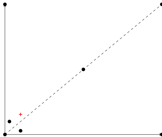
(d) RecLMTD - (3, 5, 2)
