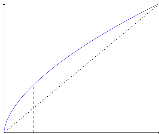
(d) q^\beta - (3, 4, 1)
