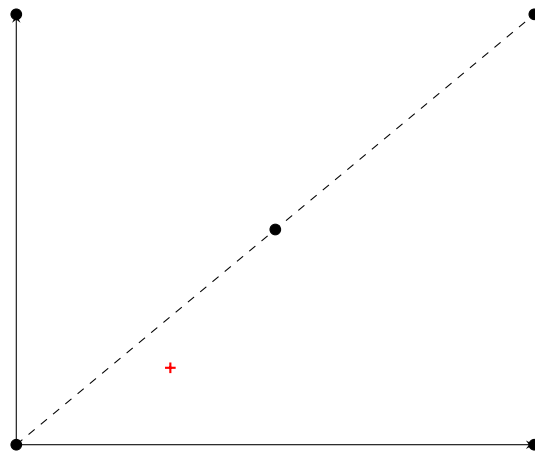
(d) RecLMTD - (3, 4, 1)
