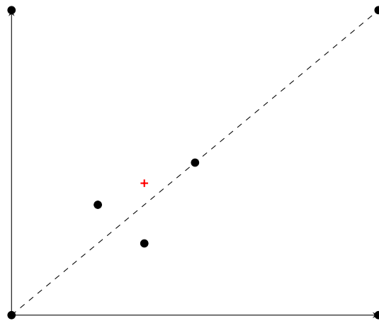
(d) RecLMTD - (3, 1, 1)
