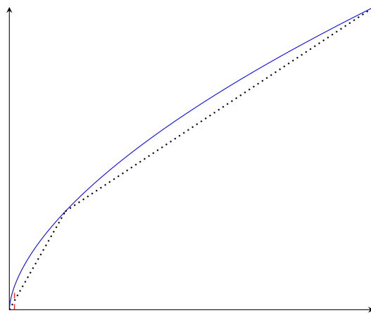
(d) q^\beta - (3, 1, 1)
