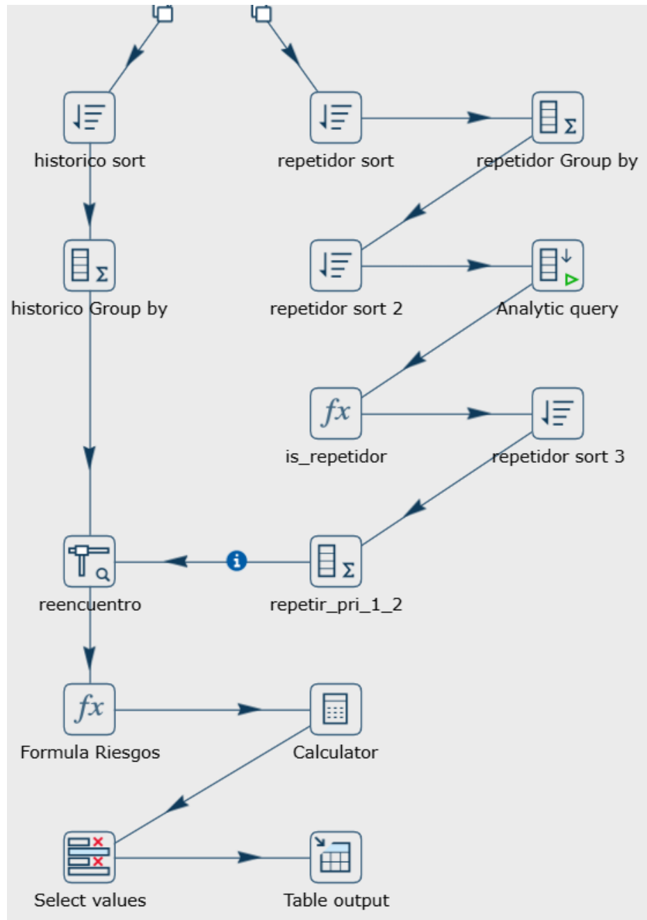
Figura 7.12: Flujo del pipeline fact_rendimiento_anual_full.hpl (Parte 2).
