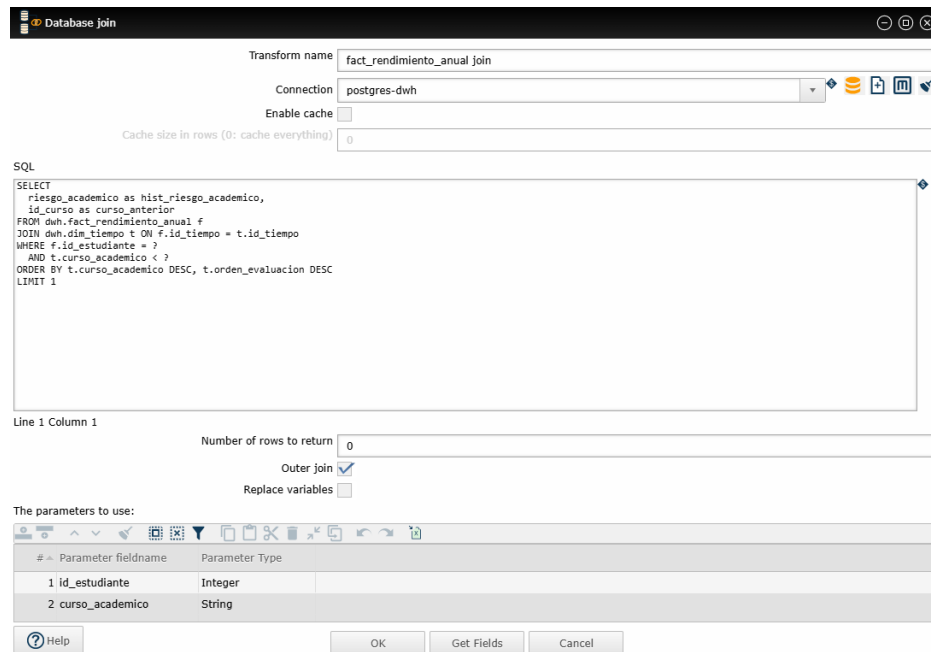
Figura 7.14: Nodo Database Join en fact_rendimiento_anual_incremental.hpl .
