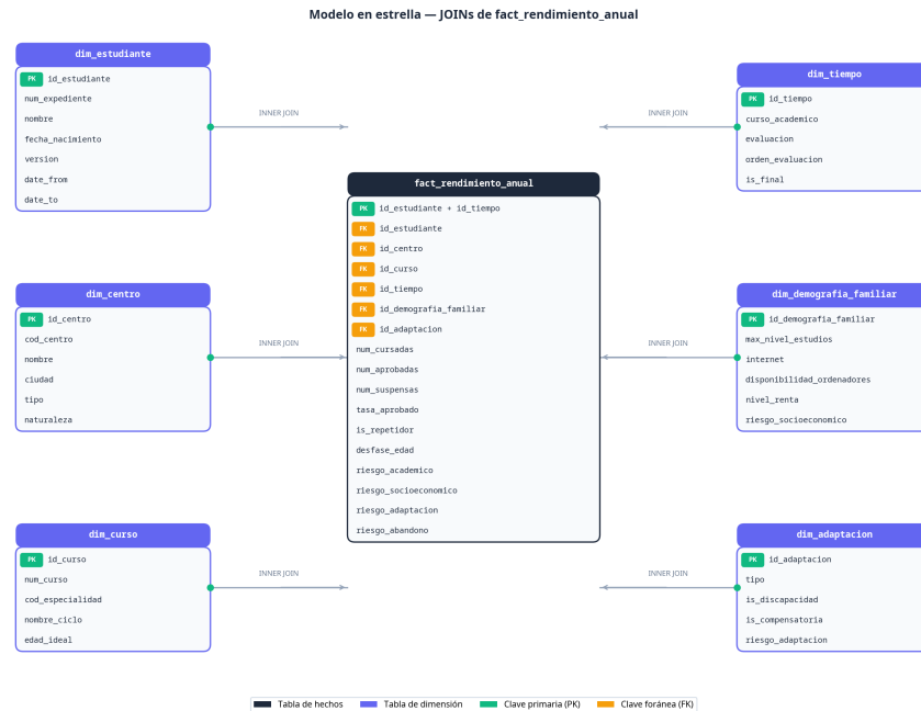
Figura 8.4: Modelo en estrella base para consultas analíticas.
