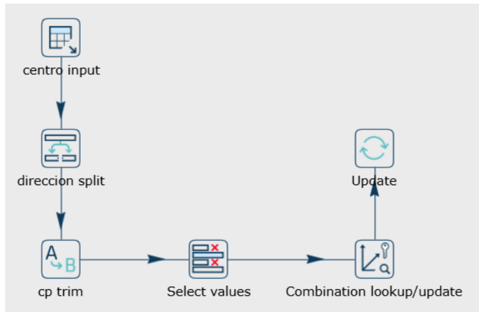
Figura 7.8: Flujo del pipeline dim_centro.hpl .
