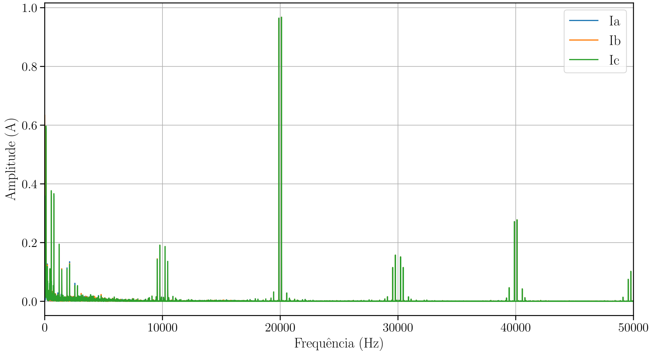
FFT das Correntes Trifásicas
