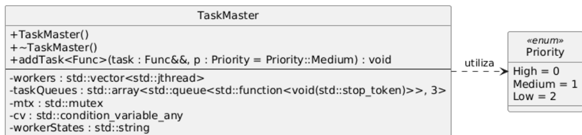
Figura 14 – Diagrama de classes da arquitetura do TaskMaster
