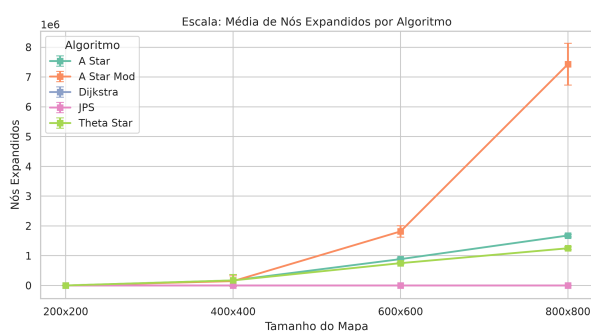
Figura 16 – Tendência de Nós Expandidos sob a variação de Escala.
