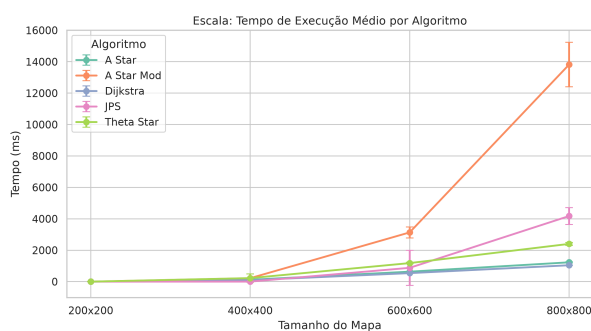
Figura 15 – Tendência de Tempo de Execução sob a variação de Escala.
