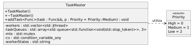
Figura 1: Diagrama de classes da arquitetura do TaskMaster
