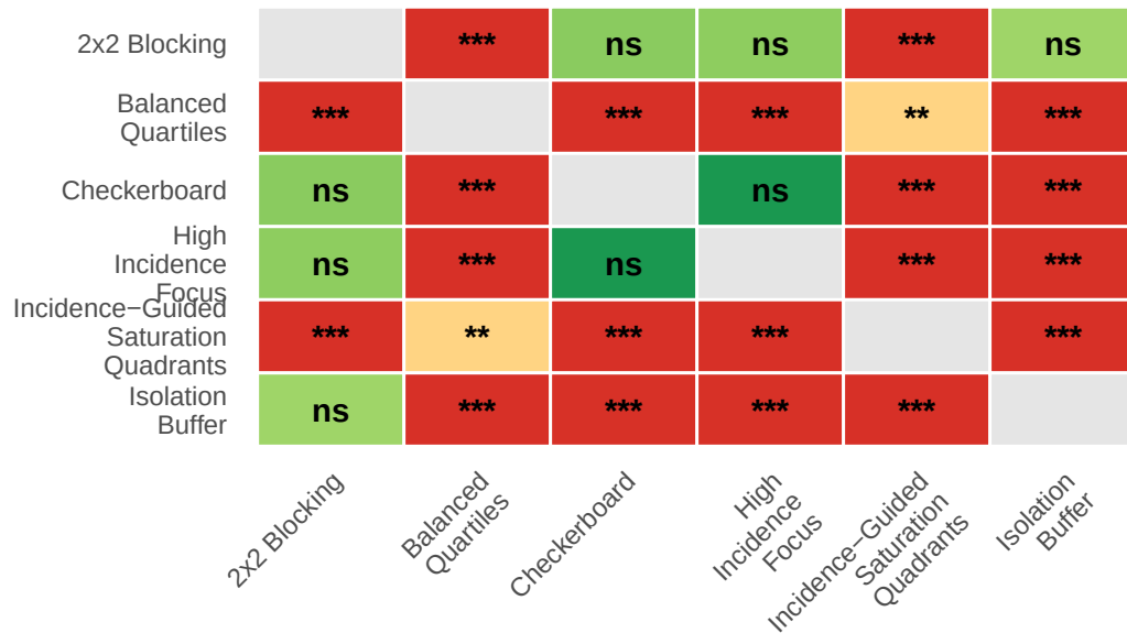
Pairwise Nemenyi p-values
