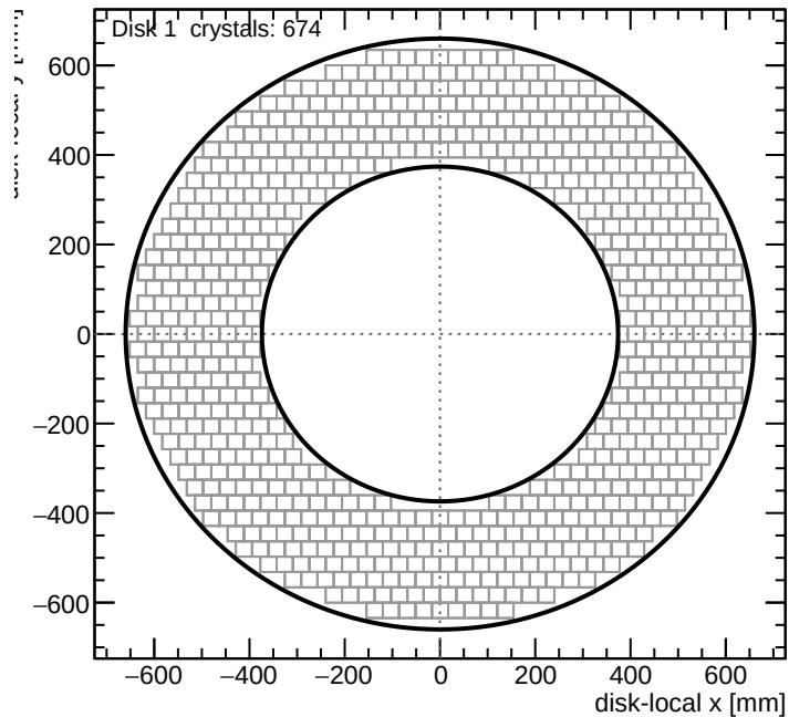
Calorimeter disk 1
