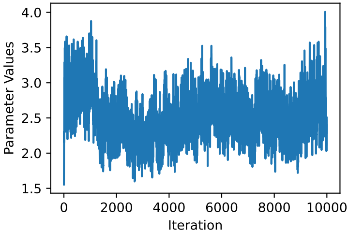
Parameter Trace: sigma2_global
