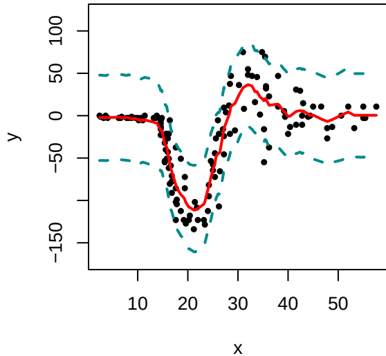
Homoskedastic BART
