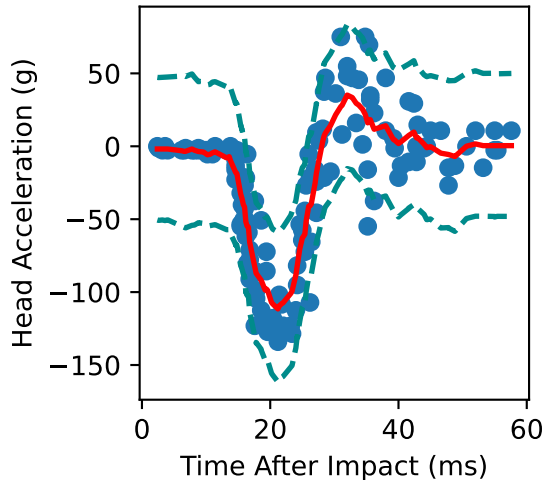
Homoskedastic BART
