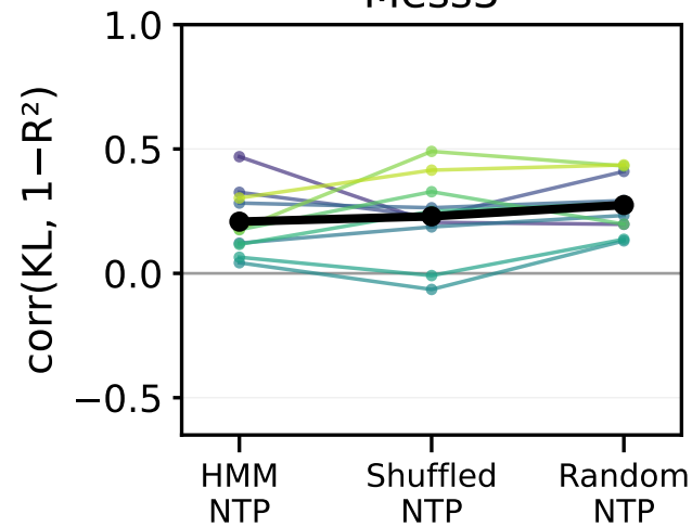
Mess3
