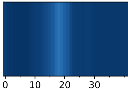
Mess3
