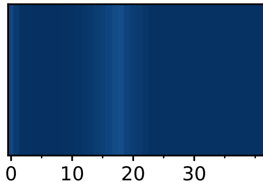
Strata
