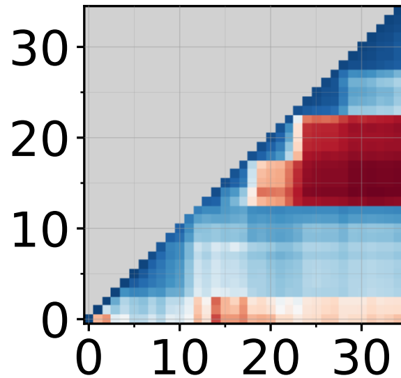
Mess3
