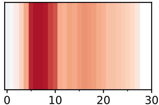
Mess3
