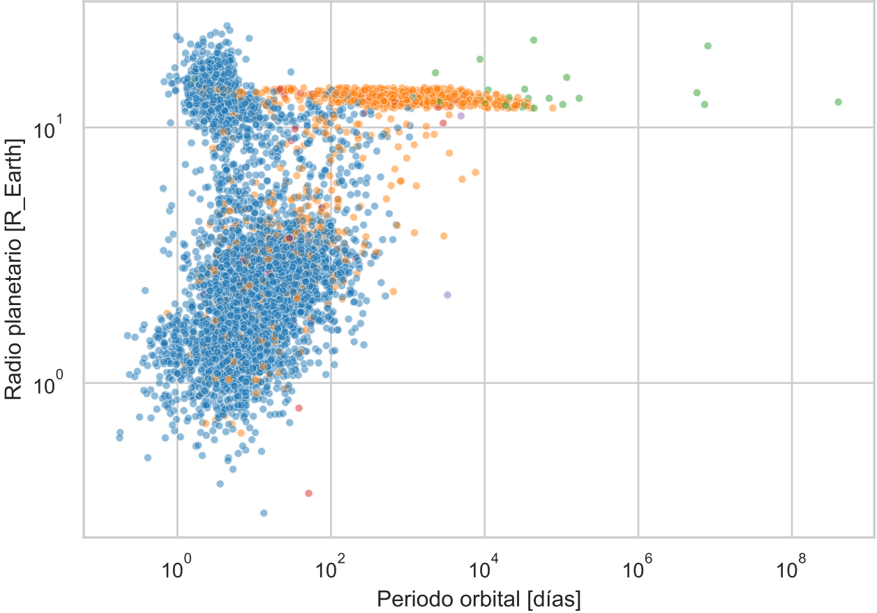
Diagrama Periodo-Radio
