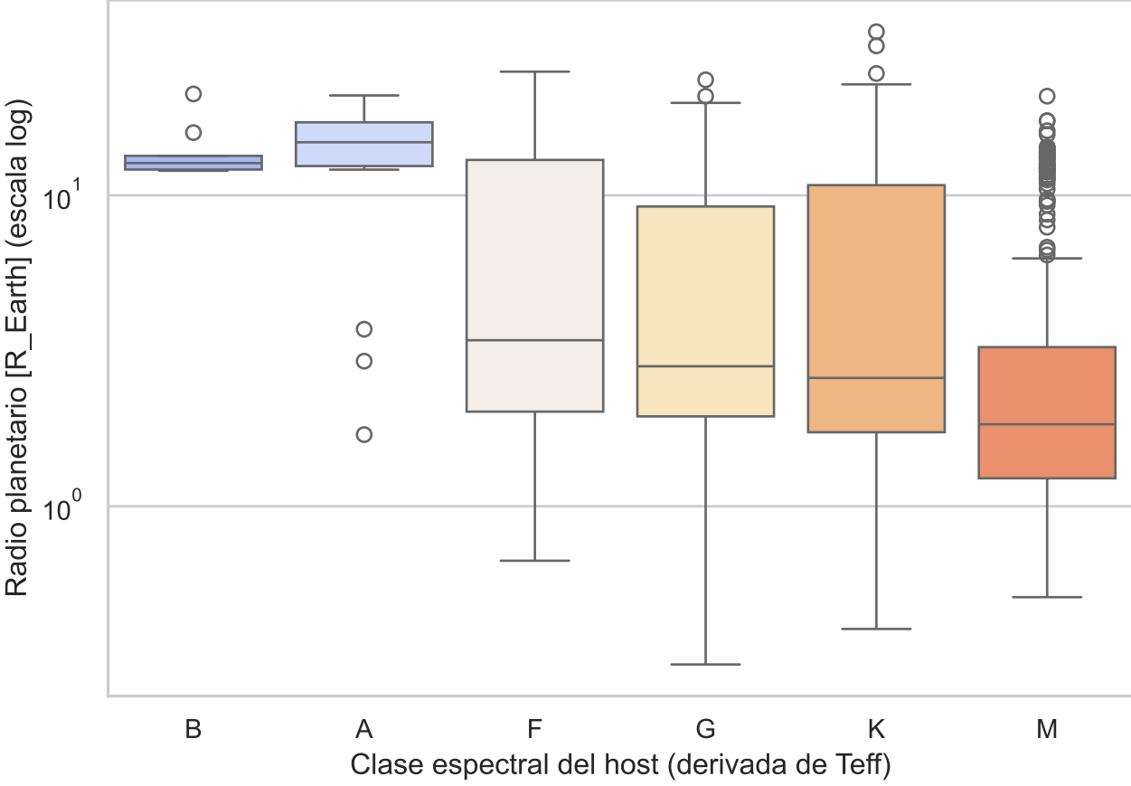
Radio planetario por tipo de estrella host
