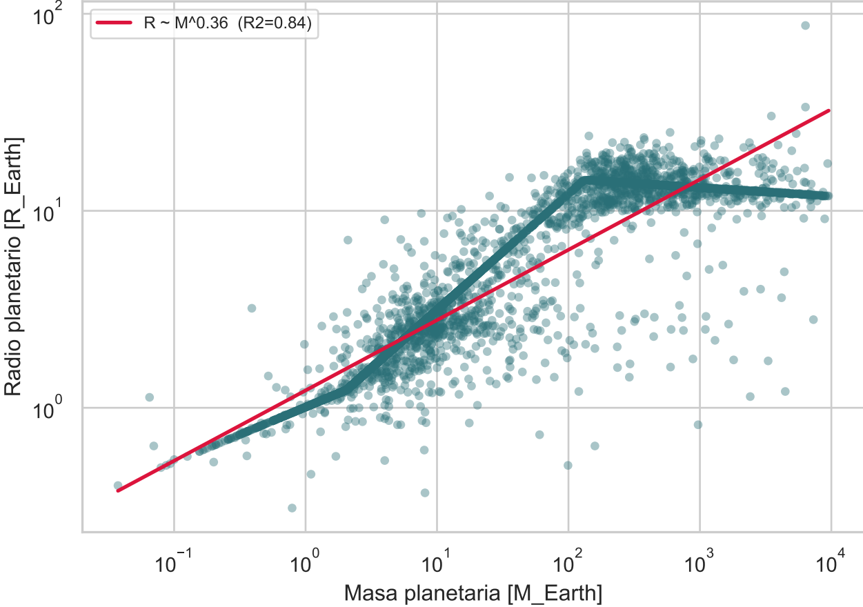
Relación Masa-Radio
