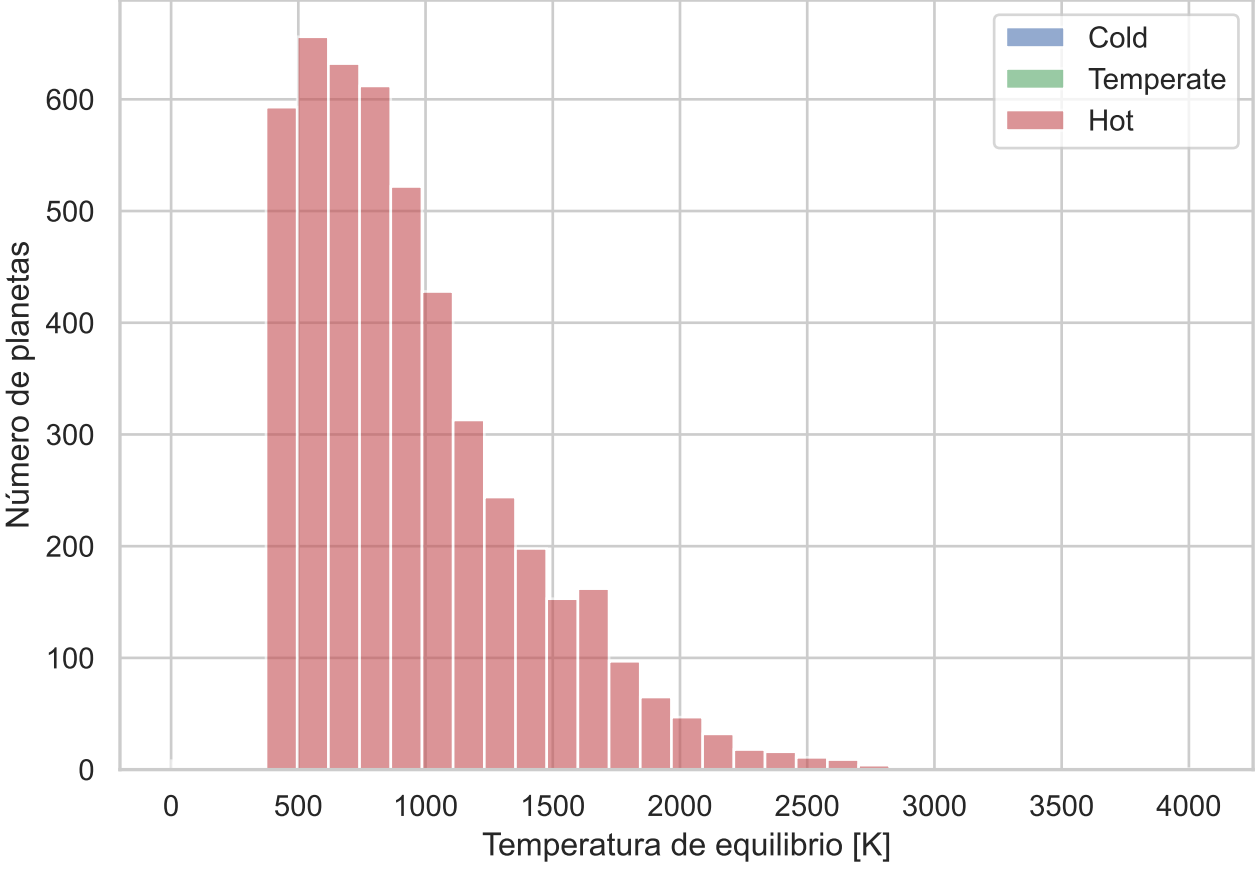
Temperatura de equilibrio (coloreado por zona)
