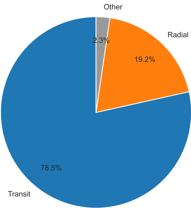
Distribución por método de detección
