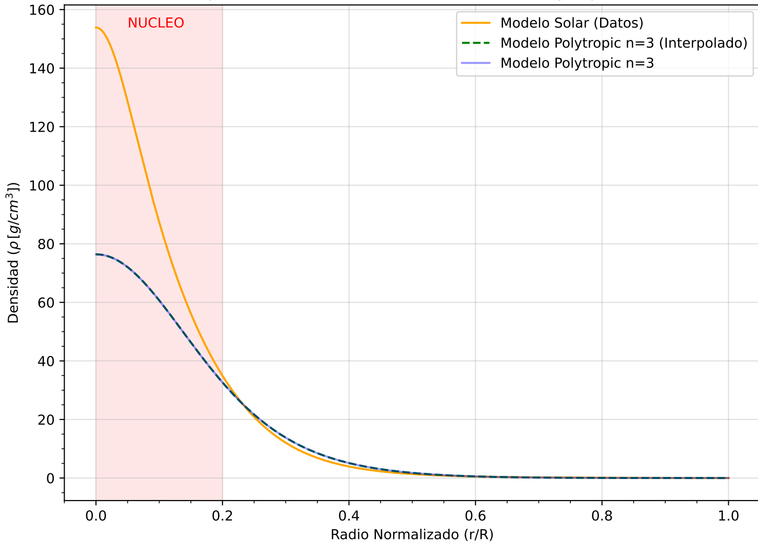
Comparación de Densidad: Modelo Solar vs Polytropic n=3
