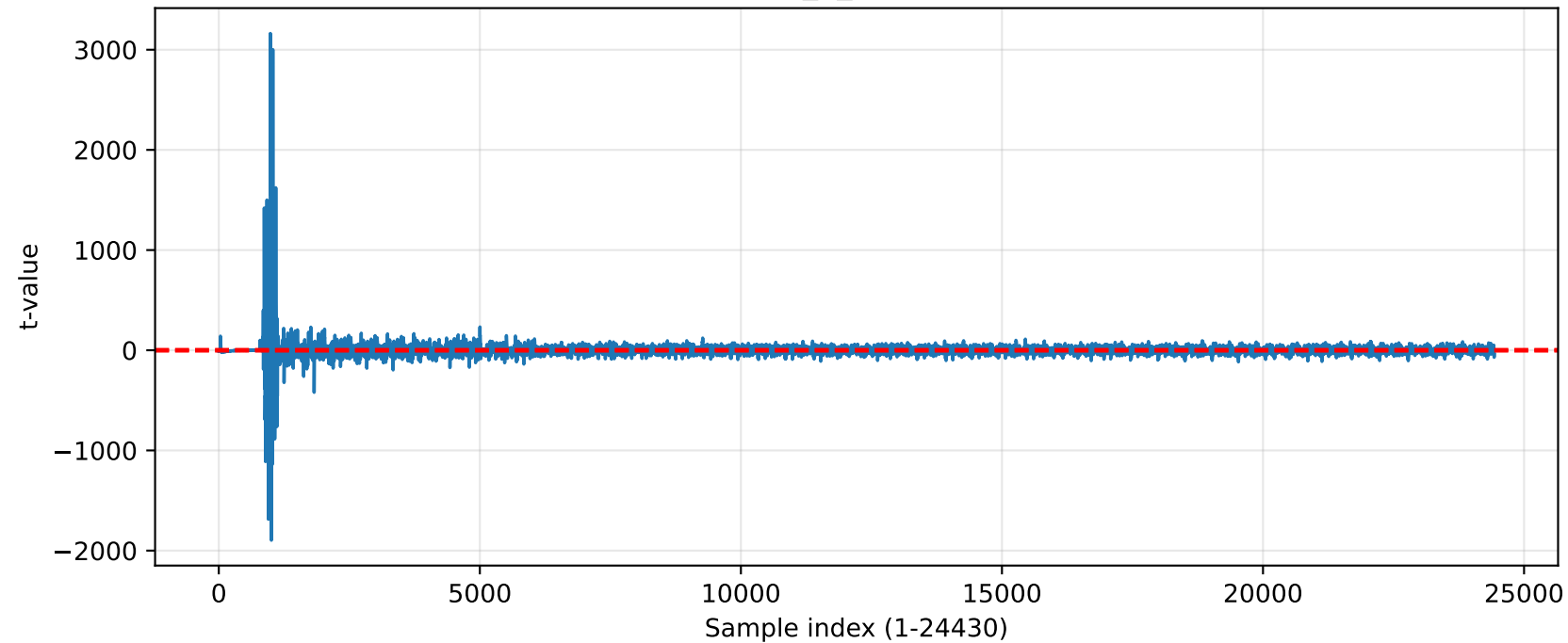
TVLA — unprotected_2_neuron (exceed=21813)
