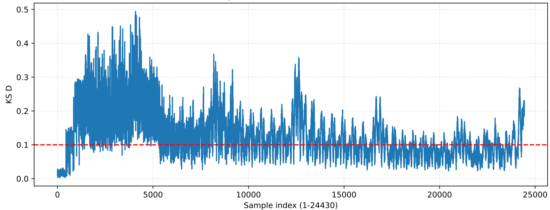
KSLA — protected1neuron (exceed=14193)
