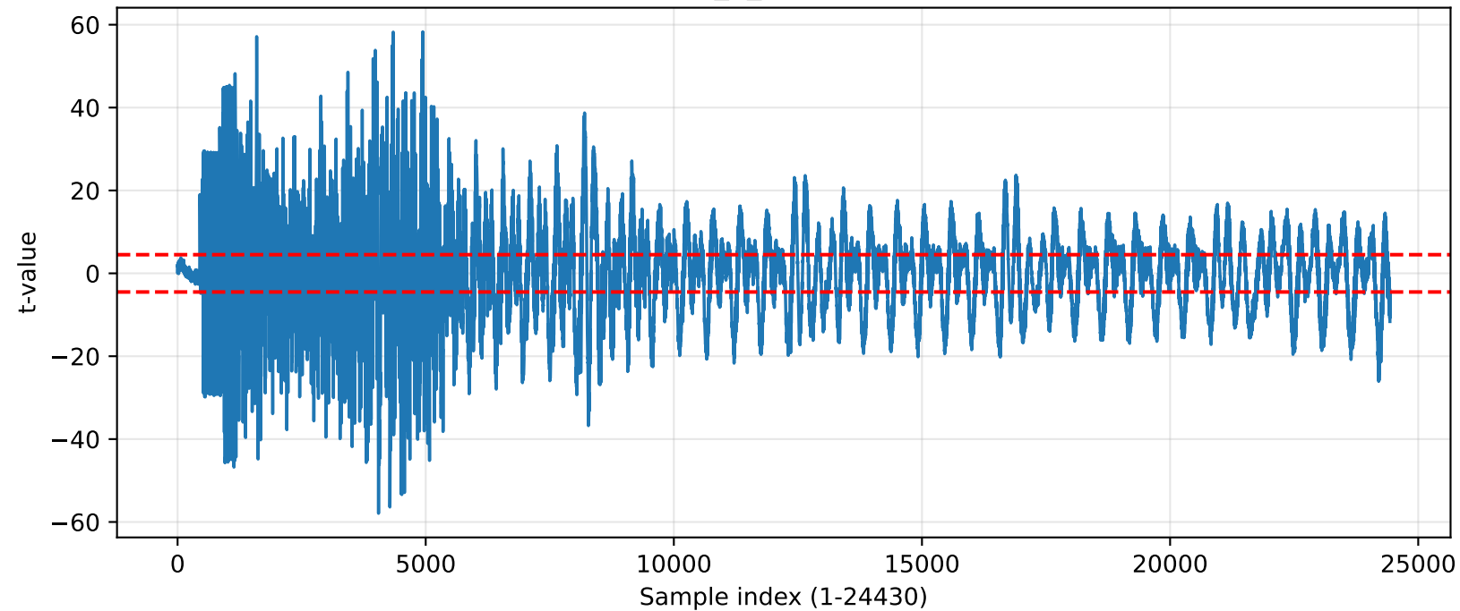
TVLA — protected_2_neuron (exceed=15861)
