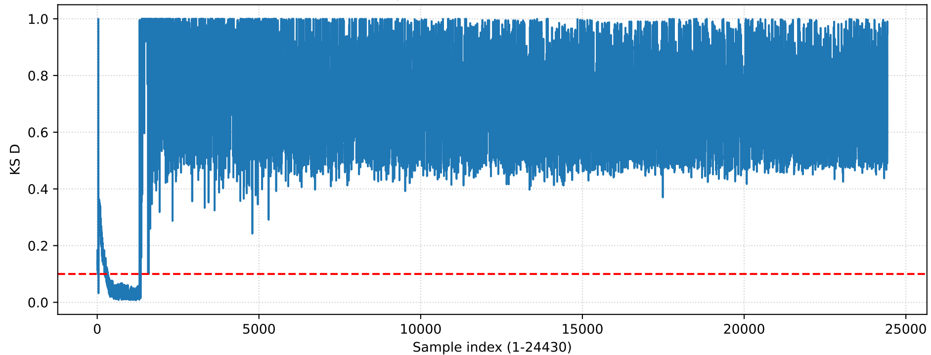
KSLA — unprotected3neuron (exceed=23394)
