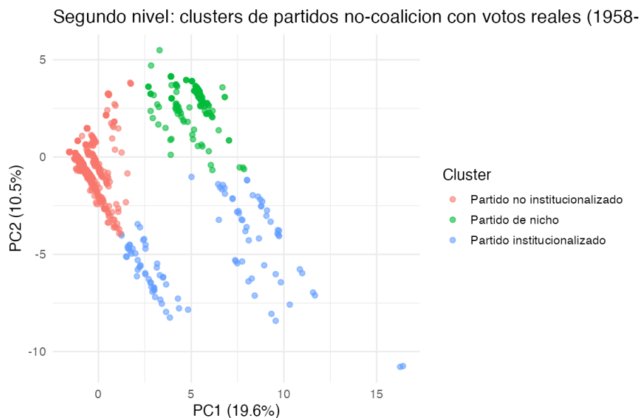
Figura 3: Segundo nivel: clusters de partidos no-coalición con votos electorales reales, proyectados sobre PCA.
