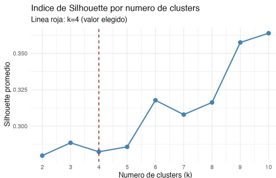
Figura 1: Índice de silhouette por número de clusters (línea punteada: k = 4 , valor elegido).
