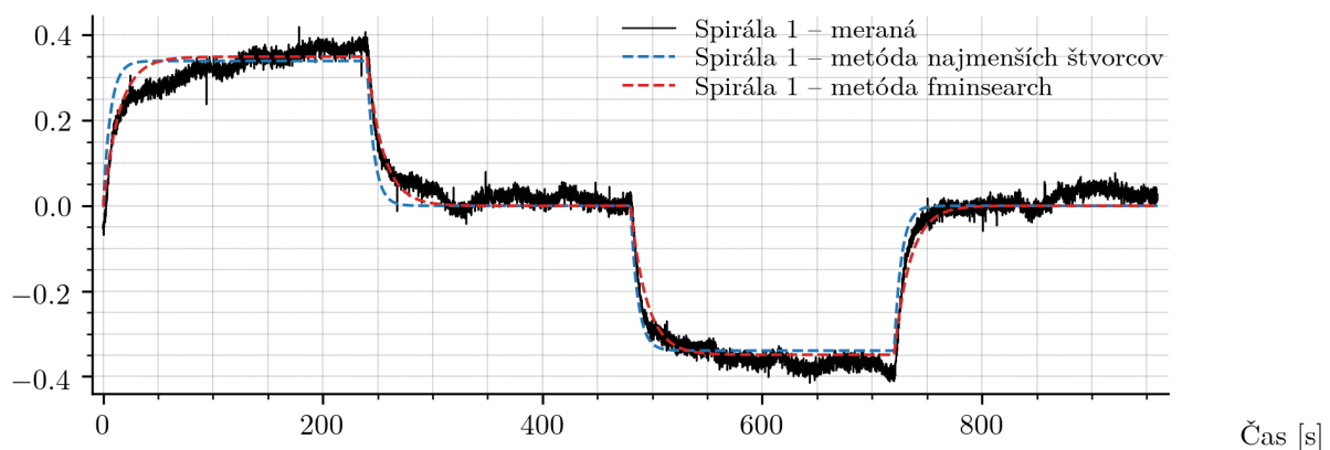
Obr. 13: Porovnanie skokovej odozvy reálneho systému TSo5 a identifikovaných modelov
