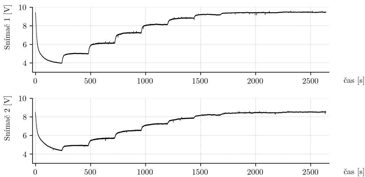
Obr. 4: Odozva systému TS05 pre pracovný bod ventilátora 3 V
