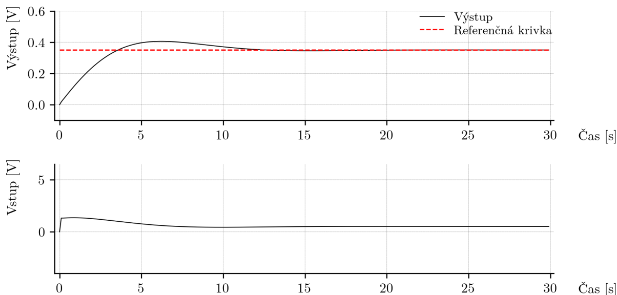
Obr. 16: Simulačný výsledok uzavretého PI riadenia systému TS05
