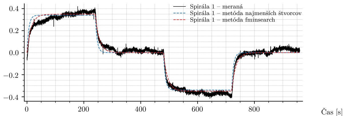
Obr. 14: Porovnanie skokovej odozvy reálneho systému TSo5 a aproximovaných modelov
