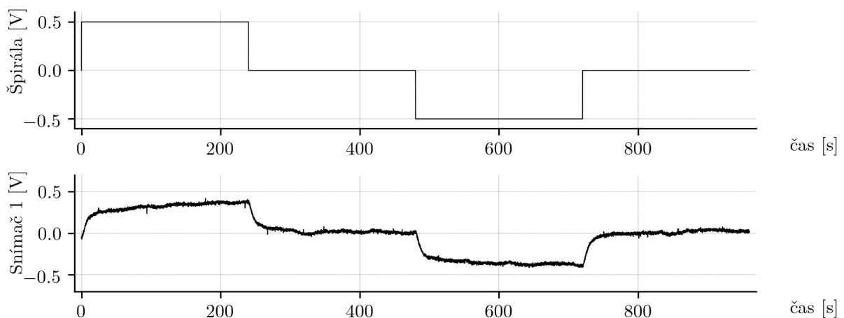
Obr. 13: Priemerná odozva systému TS05 v pracovnom bode 4 V
