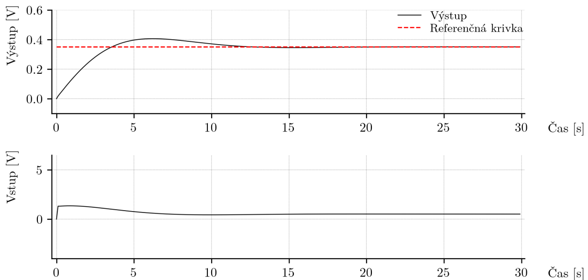
Obr. 16: Simulačný výsledok uzavretého PI riadenia systému TS05
