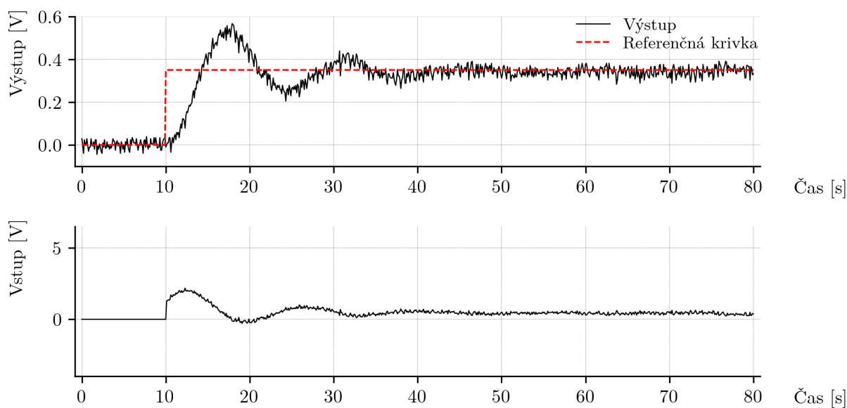
Obr. 18: Simulačný experiment s PI regulátorom pri skokovej zmene žiadanej hodnoty
