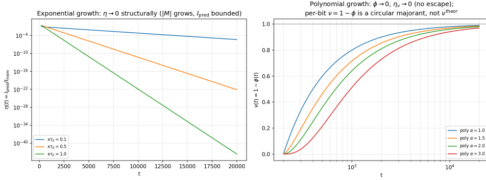
Рис. S5. Серия superlinear_memory , экспоненциальный побег и структурная малость \eta_v . При |M_{\leq t}| = M_0 e^{\kappa t} доля свежих выходит на ненулевой предел \varphi_\infty = 1 - e^{-\kappa \tau_E} \in \{0,095; 0,394; 0,632\} (побег: \nu^{\text{theor}} < 1 ), но удерживаемая ёмкость раздувается до |M_{\leq t}|(T)/|M_{\leq t}|(0) до 9,8 \cdot 10^{42} ; знаменатель I_{\text{mem}} растёт неограниченно ( \leq H(X_E^{\leq t}) , \sim линейно; в прогоне взят \propto |M_{\leq t}| как консервативная оценка) при горизонт-ограниченном I_{\text{pred}} \leq H_\tau , так что \eta_v \rightarrow 0 структурно (ёмкостно-оценочное \eta_v(T)/\eta_v(0) до 1,0 \cdot 10^{-43} ; истинный спад \sim 1/t ). Побег формально удерживает \nu^{\text{theor}} ниже 1, но информационно — память \gg предсказание, и \eta_v ничтожна. Коллапс \eta_v — структурный (рост знаменателя), не энергобюджетная расходимость.
