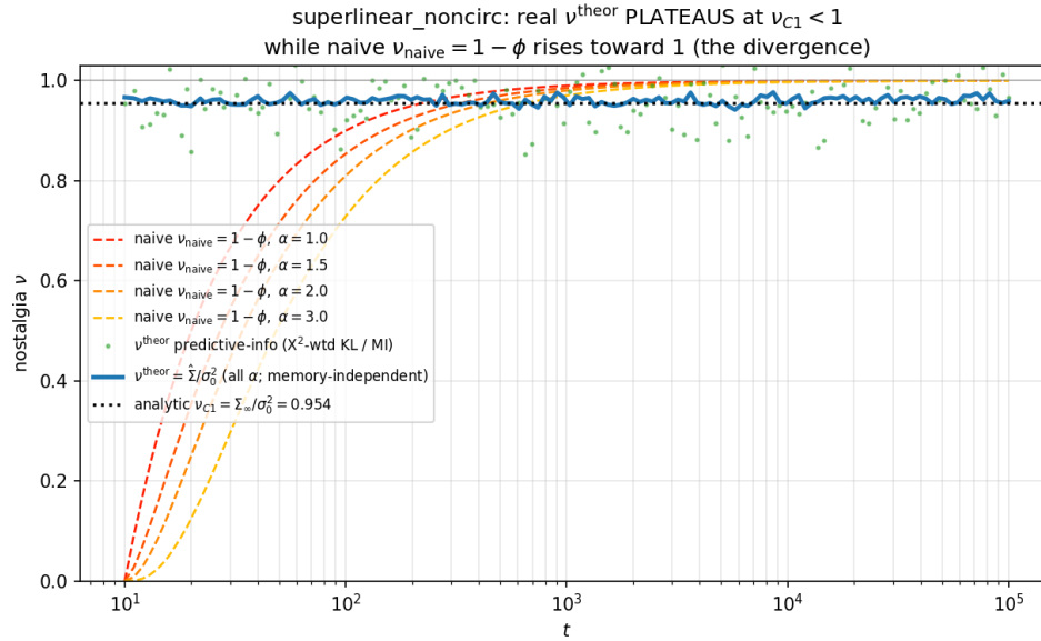
Рис. S6. Серия superlinear_noncirc : плато \nu^{\text{theor}} у пола C1 и расхождение с наивным мажорантом. Первичная (Фишер-сокращённая) \nu^{\text{theor}} = \hat{\Sigma}/\sigma_0^2 (сплошная) выходит на плоское плато \approx 0,96 , совпадающее с аналитическим \nu_{C1} = \Sigma_\infty/\sigma_0^2 = 0,954 (пунктир), \alpha -независимо; альтернативная predictive-info мера (точки) рассеяна вокруг того же уровня. Наивная per-bit-мажоранта \nu_{\text{naive}} = 1 - \phi (штриховые, \alpha \in \{1; 1,5; 2; 3\} ) вместо этого ползёт к 1 — циркулярный артефакт пороговой модели superlinear_memory (§ S4.4). Расхождение сплошной и штриховых — несущее свидетельство: реальная \nu^{\text{theor}} стоит у \nu_{C1} < 1 , а не насыщается к 1.
