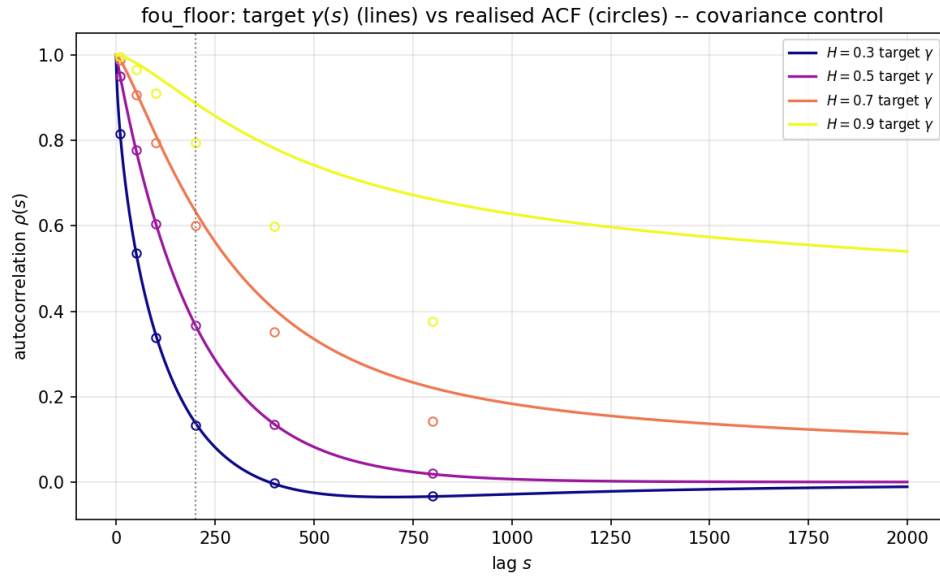
Рис. S3. Серия fou_floor , контроль ковариации. Эмпирическая лаг-корреляция реализованных путей \hat{\rho}(s) против целевой \gamma(s) : совпадение (отн. ошибка < 5\% ) до лага \sim 200 –400, где конечновыборочный оценщик ACF несмещён; на больших лагах сам оценщик ACF на долгой памяти смещён к нулю — поэтому дальний хвост показателя читается по точной \gamma , которую пути воплощают по построению, а не по выборочной ACF. Подтверждает, что генерируется подлинный стационарный fOU.
