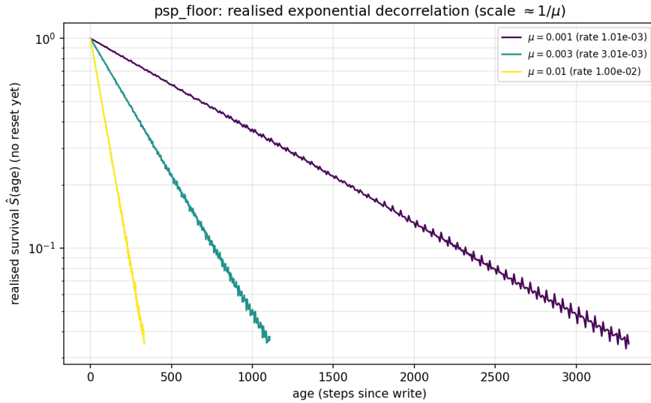
Рис. S4. Серия psp_floor , реализованная кривая выживания \hat{S}(\text{возраст}) (доля удержанных битов данного возраста, ещё не увидевших сброс) в полулогарифмических координатах. Наклон даёт скорость декорреляции 1,01 \cdot 10^{-3} , 3,01 \cdot 10^{-3} , 1,00 \cdot 10^{-2} ; каждый bootstrap-ДИ накрывает номинальный \mu = 1/\tau_E — настоящее измерение шкалы 1/\mu из реализованного процесса (равенство \mu не постулируется).
