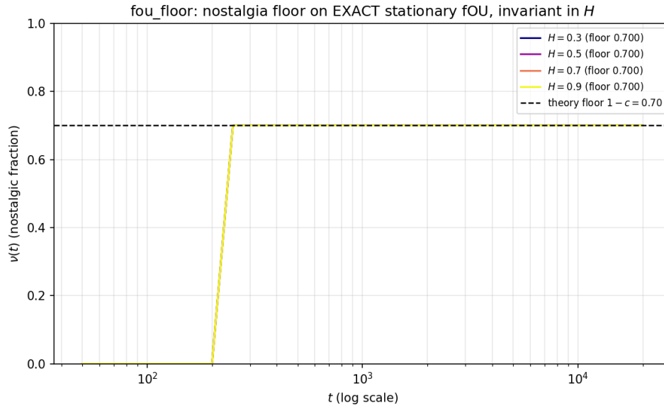
Рис. S2. Серия fou_floor , инвариантность глубины пола по H (по построению; лог-ось t ). Ностальгическая доля \nu(t) равна нулю, пока буфер моложе горизонта корреляции \tau_E = 200 (ни один бит ещё не старше \tau_E ), затем выходит на пол 1 - c = 0,700 , одинаковый для всех H \in \{0,3; 0,5; 0,7; 0,9\} — кривые совпадают (инвариантность глубины). Пол здесь зашит пороговой моделью (доля свежих = c через горизонт \hat{\rho}^2(\tau_E) ): иллюстрация инвариантности на корректных fOU-путях, а не независимое измерение — независимую оценку глубины несёт реализованный PSP-поток (рис. 3 основного текста).
