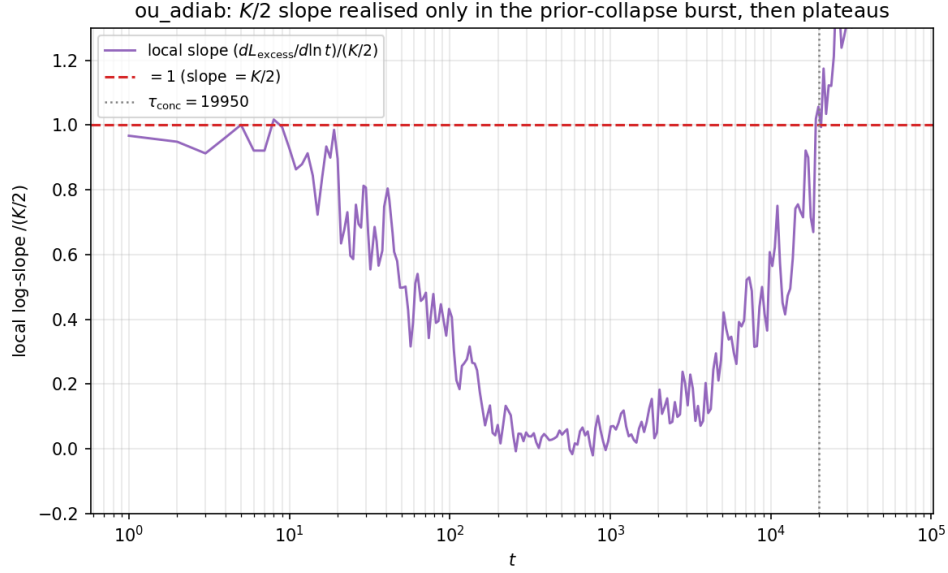
Рис. S1. Серия ou_adiab , эксперимент (В): локальный лог-наклон L_{\text{excess}} против t . Наклон равен K/2 только в коротком всплеске коллапса приора ( t \lesssim \tau_{\text{conc}} , наклон 0,936 на [1, 20] ); после него установившийся g^* ограничивает n_{\text{eff}} \approx 1/g^* , лог-компонента выходит на плато высотой \sim (K/2) \ln(1/g^*) , и наклон лог-члена падает до 0,099. Полная L_{\text{excess}} продолжает линейный рост A \cdot t — это насыщение лог-члена, не глобальный коллапс.
