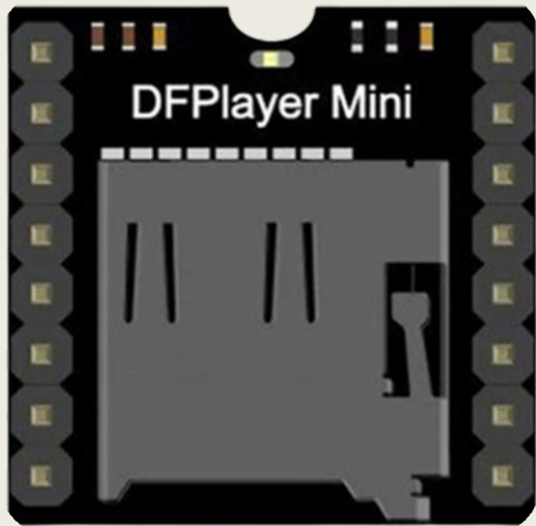
MP3-PLAYER INKL LAUTSPRECHER UART0 (TX, RX)
