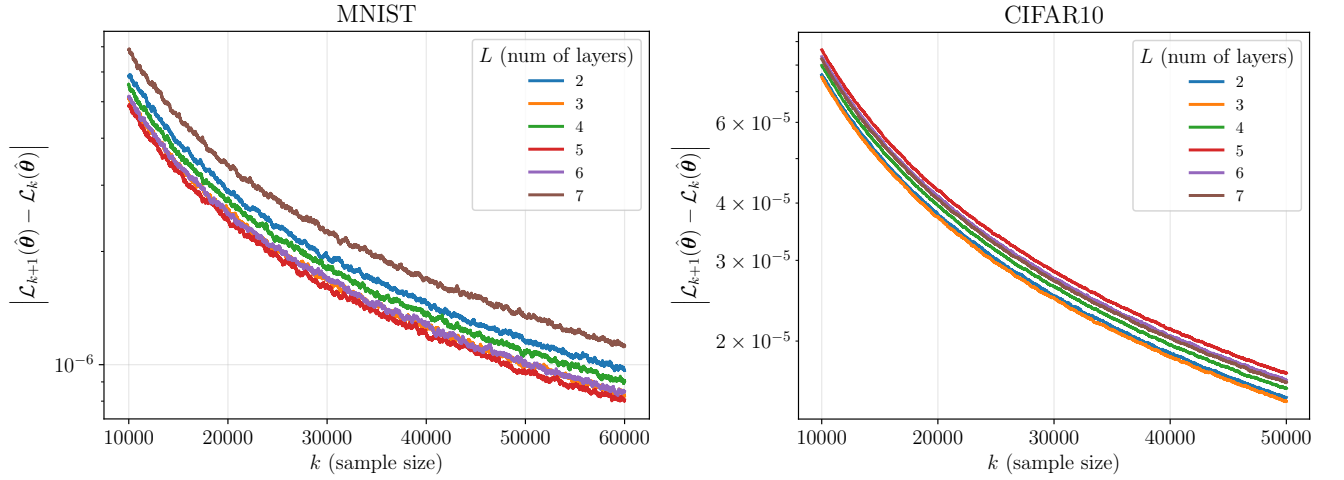
Рис. 2.20: Зависимость абсолютного значения разности функций потерь |\mathcal{L}_{k+1}(\theta) - \mathcal{L}_k(\theta)| от размера выборки k для сверточной нейронной сети при изменении количества сверточных слоев L при фиксированных размере ядра k = 3 и количестве каналов C = 6 . Графики демонстрируют немонотонный характер зависимости разности потерь от количества слоев.
