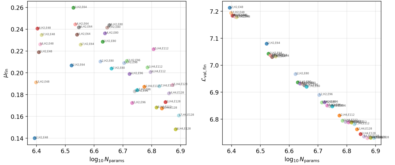
Рис. 2.13: Финальная контрольная точка первой части эксперимента: \mu и \mathcal{L}_{val} против десятичного логарифма числа обучаемых параметров N_{params} для 36 архитектур
