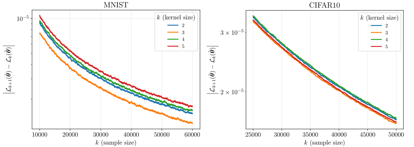
Рис. 2.21: Зависимость абсолютного значения разности функций потерь |\mathcal{L}_{k+1}(\theta) - \mathcal{L}_k(\theta)| от размера выборки k для сверточной нейронной сети при изменении размера ядра свертки k при фиксированных количестве слоев L и количестве каналов C = 6 . Графики демонстрируют немонотонный характер зависимости разности потерь от размера ядра.
