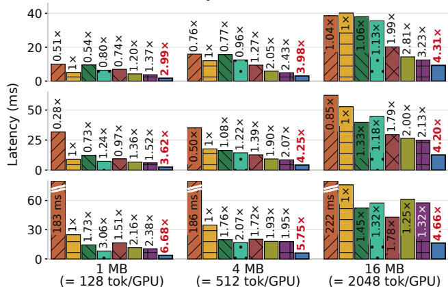
Qwen3-235B
