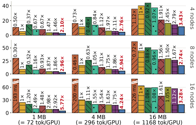
Kimi K2
