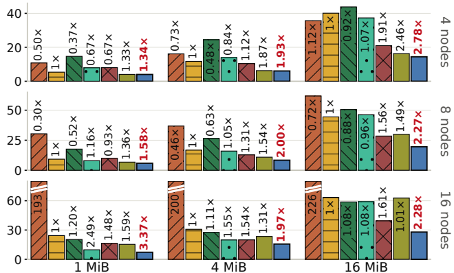
Kimi K2
