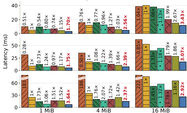
Qwen3-235B
