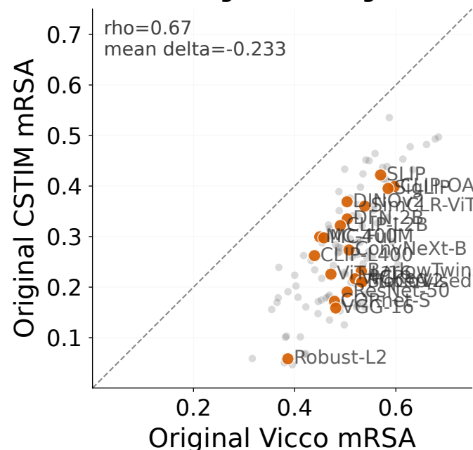
CSTIM shift
