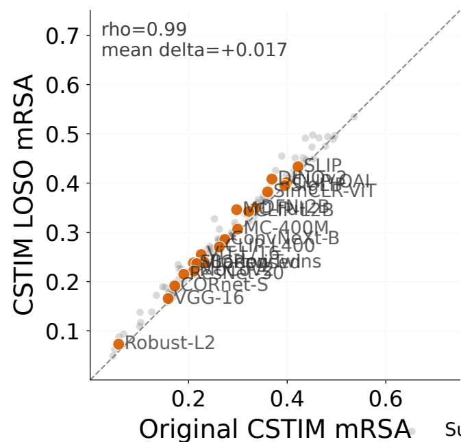
CSTIM shift
