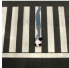
openclip_vit_so400m_14_siglip_webli query
