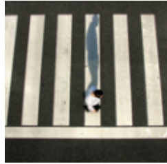
slip_vit_l_slip query
