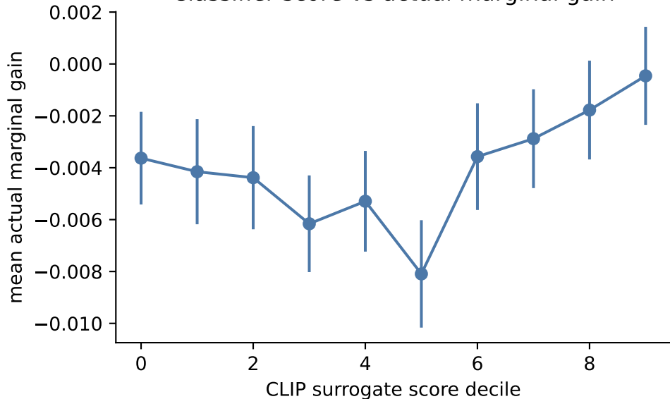
Classifier score vs actual marginal gain
