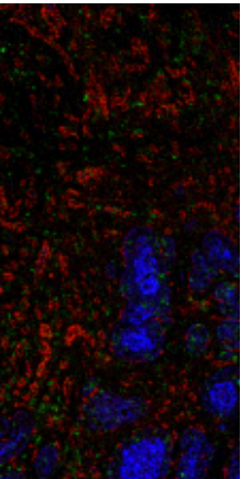
F1 ROI OC12_003 R=CD31 G=Ki-67 B=panCK (raw, 0.99-norm)
