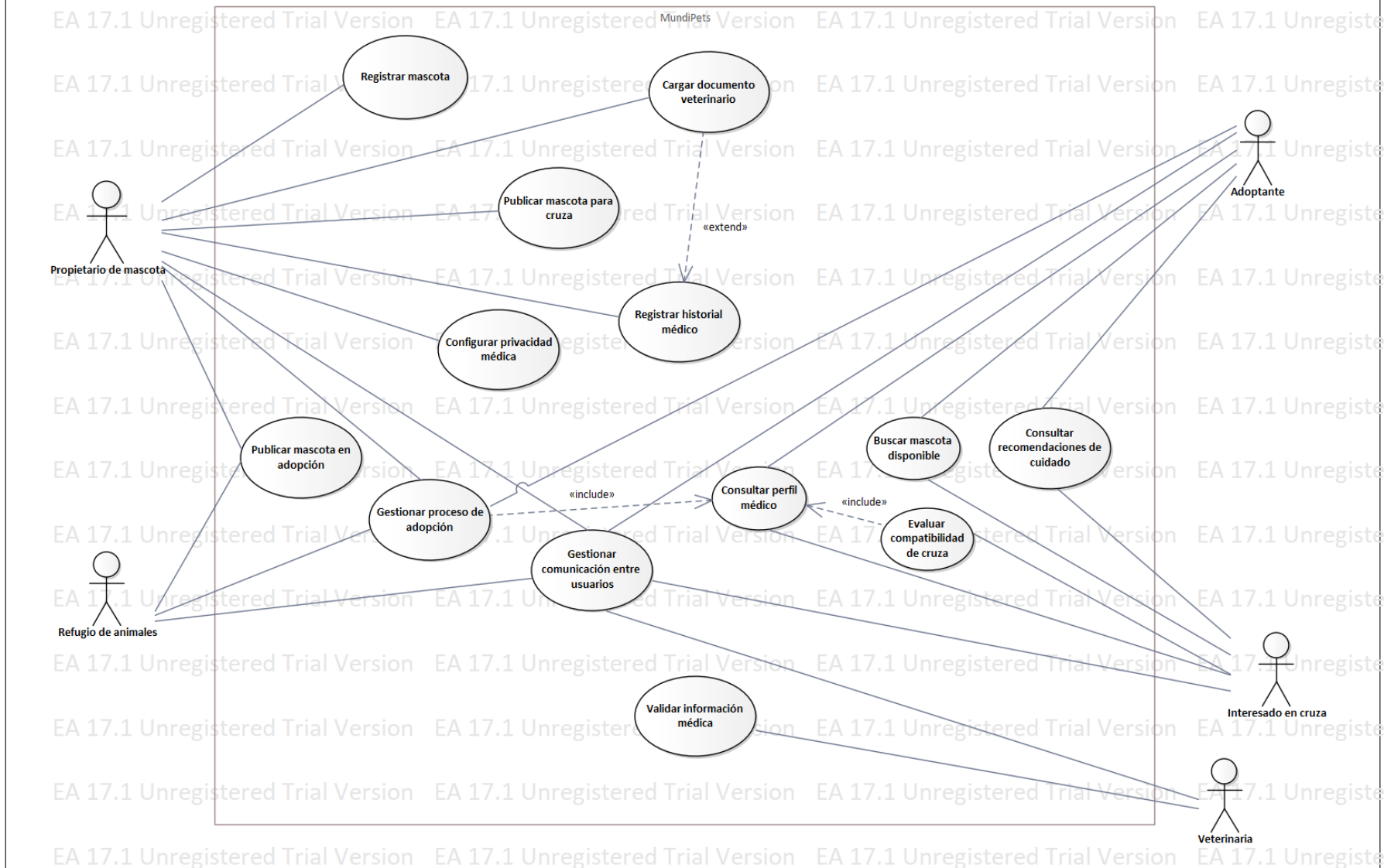
Figura 4. Diagrama de casos de uso del sistema MundiPets
