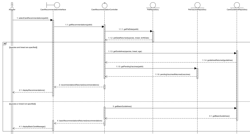
Figura 29: Diagrama de secuencia — Consultar recomendaciones de cuidado (archivo etiquetado CU-12).
