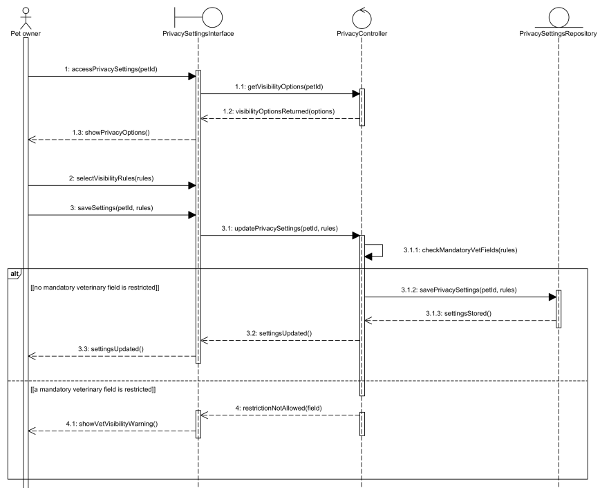
Figura 23: Diagrama de secuencia — Configurar privacidad médica (archivo etiquetado CU-06; corresponde a CU-12).
