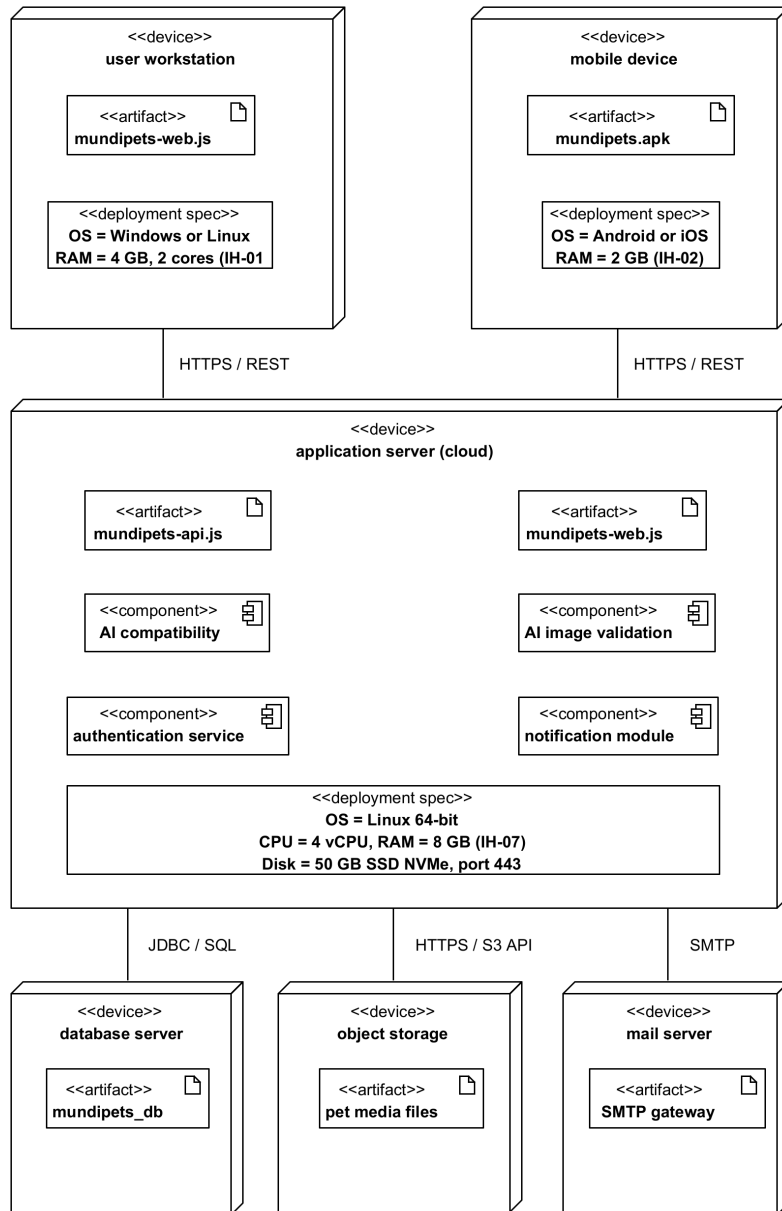
Figura 48: Diagrama de despliegue del sistema MundiPets.
