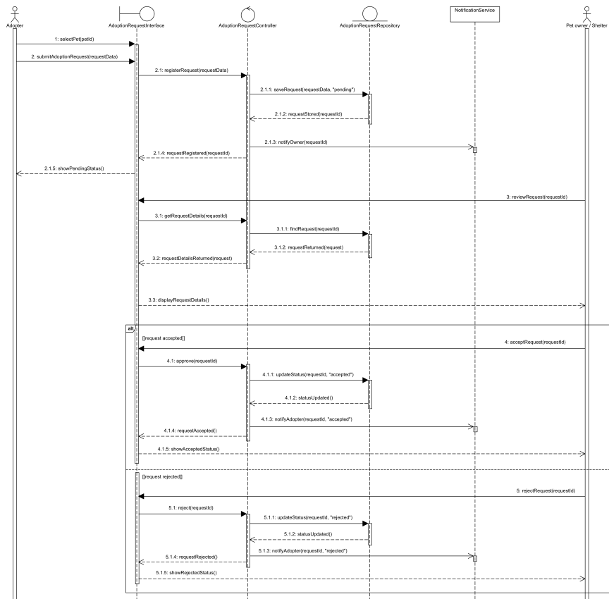
Figura 24: Diagrama de secuencia — Gestionar solicitud de adopción (archivo etiquetado CU-07).
