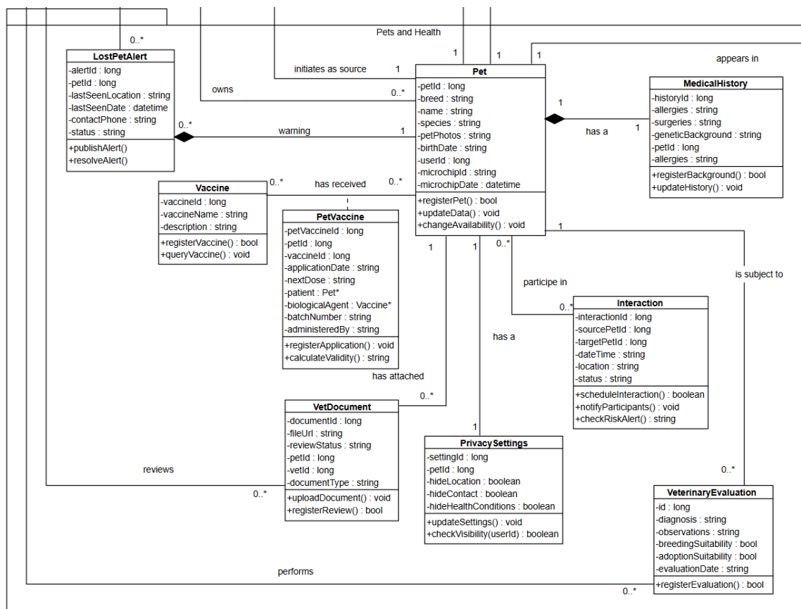
Figura 17: Diagrama de clases refinado — vista parcial Pets and Health , ya con la corrección de modelado de RF-21, RF-24 y RF-25 incorporada.
