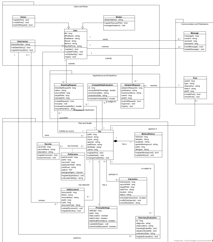
Figura 13: Diagrama de clases refinado del sistema MundiPets (vista general, previa a la corrección de modelado de RF-21, RF-24 y RF-25).
