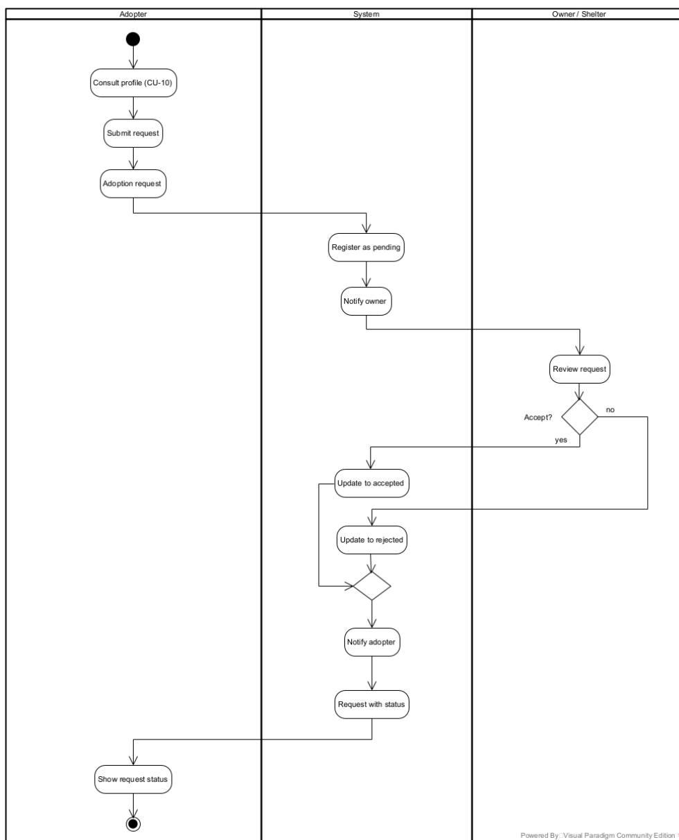
Figura 37: Diagrama de actividad — Gestionar solicitud de adopción (archivo etiquetado CU-07).
