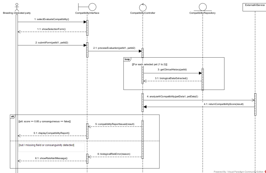
Figura 30: Diagrama de secuencia — Evaluar compatibilidad de cruce y verificación de parentesco (archivo etiquetado CU-13; corresponde a CU-06 y CU-13).
