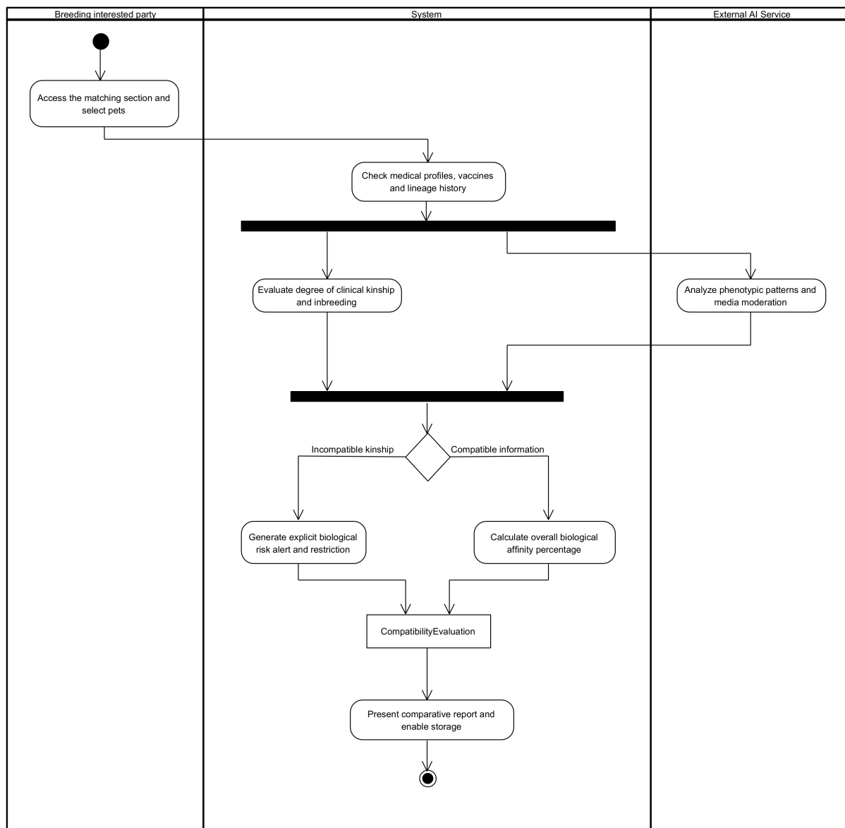
Figura 43: Diagrama de actividad — Evaluar compatibilidad de cruce y verificación de parentesco (archivo etiquetado CU-13; corresponde a CU-06 y CU-13).
