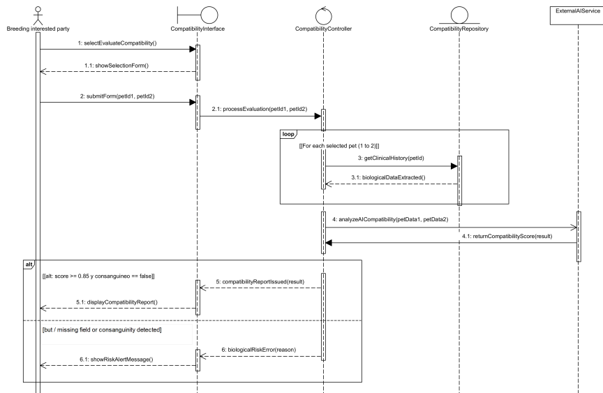
Figura 26: Diagrama de secuencia del caso de uso CU-13 — Verificación de parentesco previa a la evaluación de compatibilidad.
