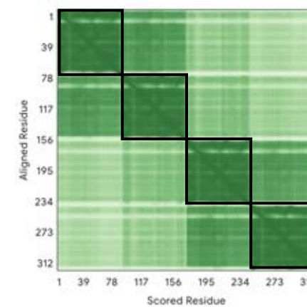
Tetramer (n=4)
