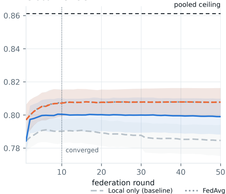
Global AUROC
