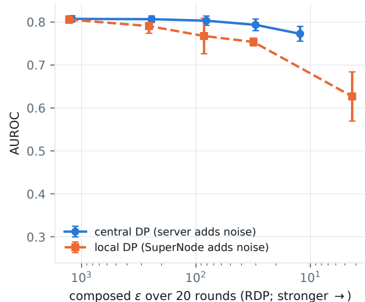
Global AUROC
