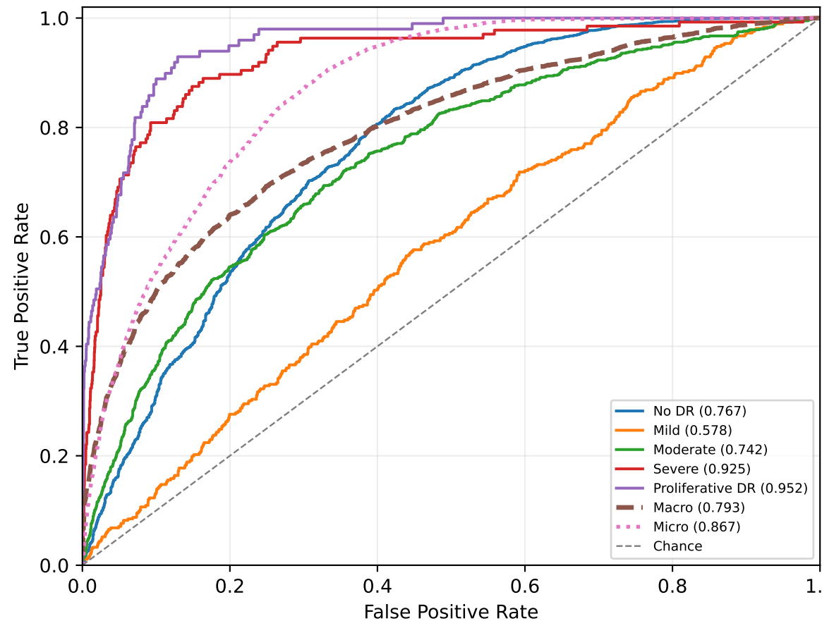
(a) EfficientNet-B4
