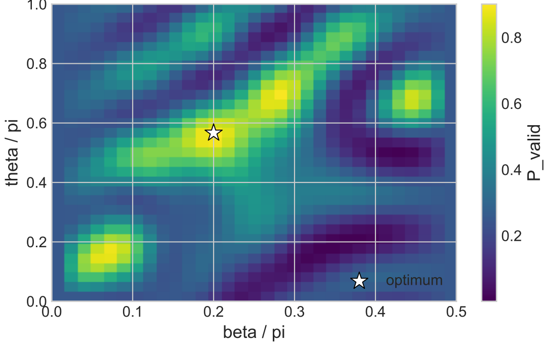
V4 P_valid heatmap at r=7 - 06_2d_tiny_corner_block
