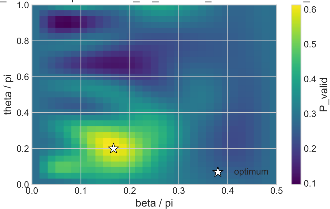
V5 P_valid heatmap at r=4 - 04_1d_clustered_medium - oriented_valid
