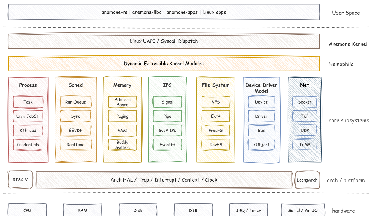
图 2 Anemone 整体架构图。
