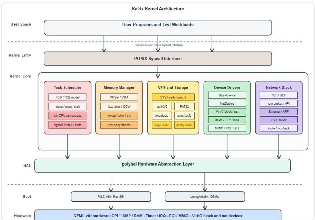
图 1-1: 总体架构
