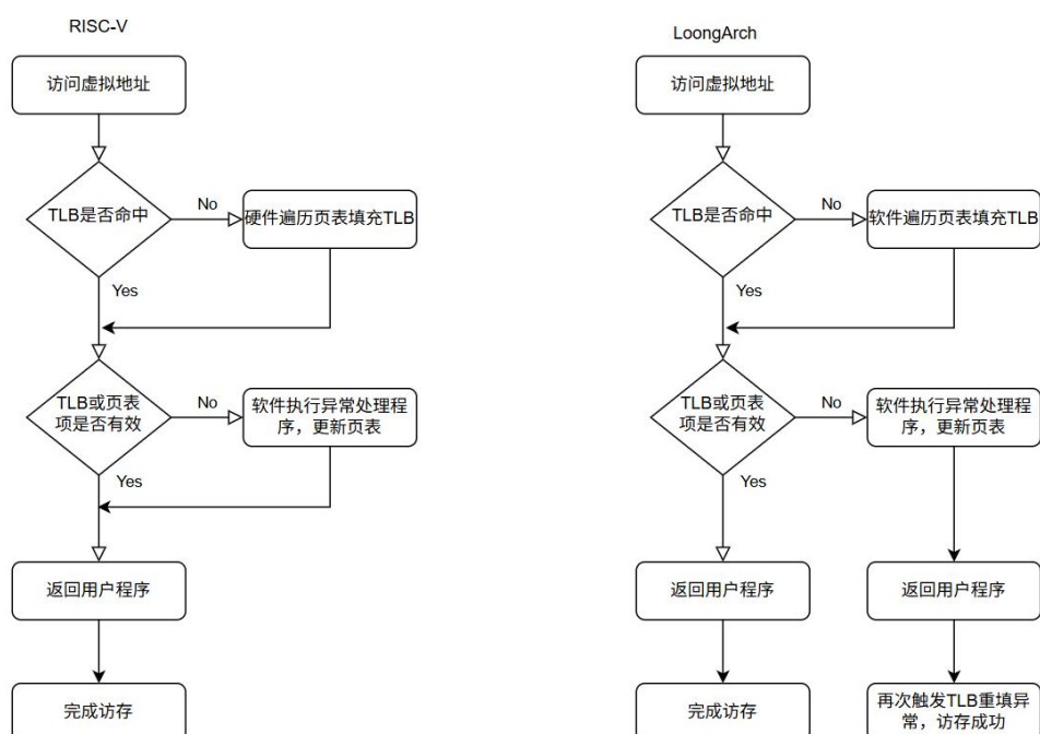
图? . RISC-V和LoongArch的异常处理路径
