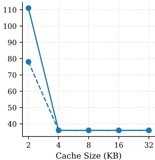
Hotspot
