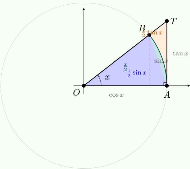
Figura 4.3: Comparación de áreas: triángulo inscrito \subset sector \subset triángulo circunscrito.
