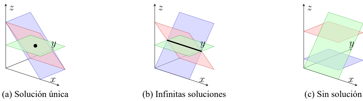
Figura 14.4: Configuraciones de tres planos en \mathbb{R}^3 según el tipo de solución del sistema 3 \times 3 : (a) los tres planos se cortan en un único punto (sistema con solución única); (b) los tres planos comparten una recta (infinitas soluciones); (c) dos planos paralelos y un tercero que los corta: no existe punto común a los tres (sistema inconsistente).
