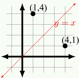
Figura 23.11: Reflexión respecto a la recta y = x .
