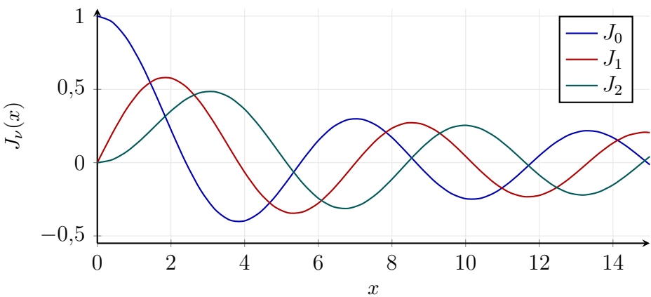
Figura 29.2: Funciones de Bessel de primera especie J_0, J_1, J_2 . Oscilan con amplitud decreciente ( \sim x^{-1/2} ); sus infinitos ceros determinan las frecuencias propias en problemas con simetría cilíndrica.
