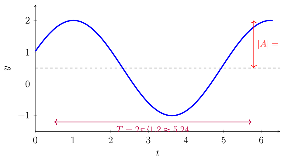
Figura 3.12: Parámetros de la forma amplitud-fase en y = C + A \operatorname{sen}[a(t - b)] .
