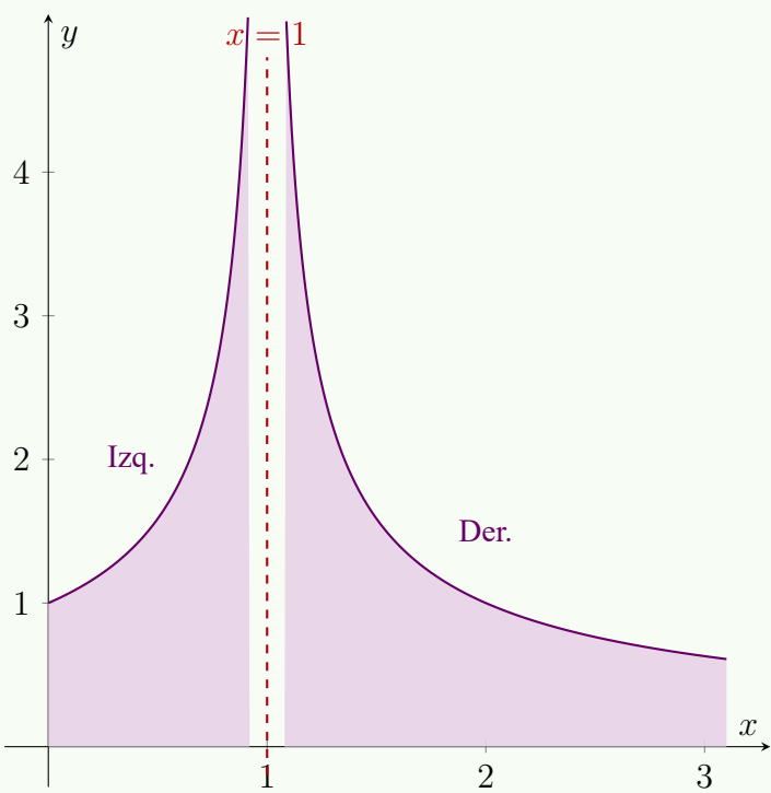
Figura 11.7: Integrando con cúspide vertical asintótica en x = 1 : es obligatorio separar la integral en [0, 1) (Izq.) y (1, 3] (Der.), pues aplicar el TFC a través de la discontinuidad da un resultado erróneo.
