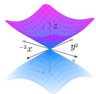
Figura 17.14: Cono circular z^2 = x^2 + y^2 , con ambas napas.
