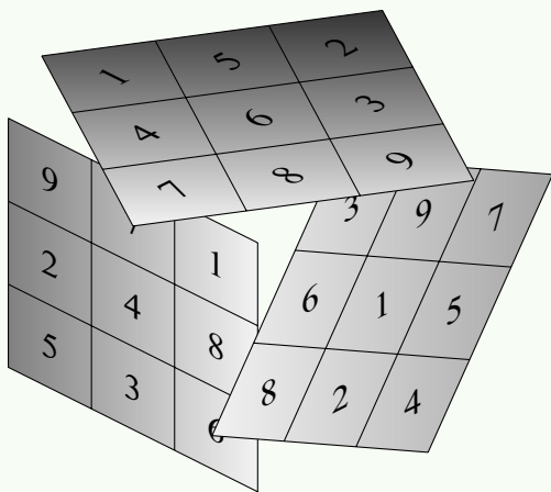
Figura 23.22: Rotación de 30° en el plano YZ alrededor del eje x.
