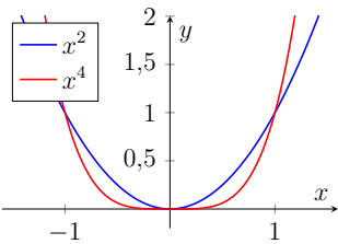
Figura 3.5: Izquierda: potencias pares (simétricas respecto al eje y ; x^4 más achatada cerca del origen que x^2 ). Derecha: potencias impares (simétricas respecto al origen).
