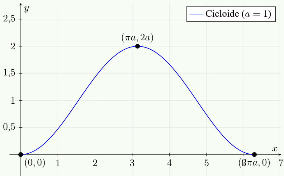
Figura 12.4: Un arco de cicloide: parte del origen en t = 0 , alcanza la cúspide (\pi a, 2a) en t = \pi y regresa al eje x en (2\pi a, 0) cuando t = 2\pi .
