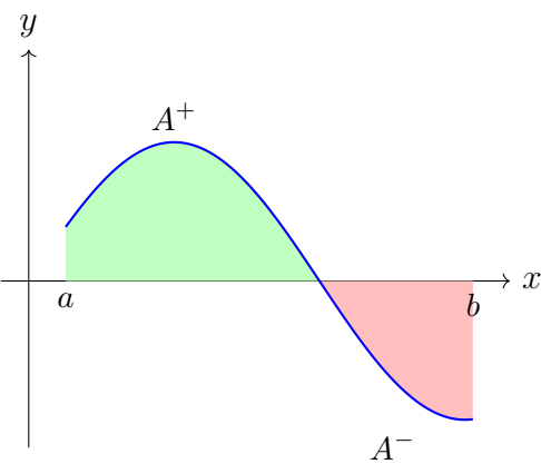
Figura 9.3: Interpretación de la integral definida como área neta : la región sobre el eje x (verde, A^+ ) aporta con signo positivo y la región bajo el eje (roja, A^- ) con signo negativo, de modo que \int_a^b f = A^+ - A^- .
