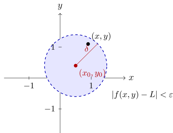
Figura 18.1: Disco abierto B((x_0, y_0), \delta) : todo punto (x, y) con 0 < \|(x, y) - (x_0, y_0)\| < \delta satisface |f(x, y) - L| < \epsilon
