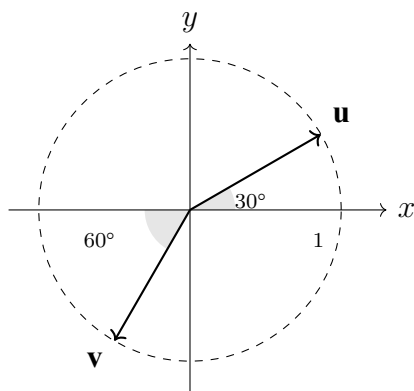
Figura 7.8: Vectores del problema 7.5
