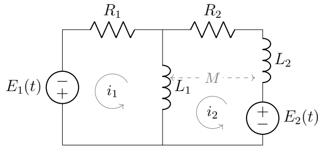
Figura 28.3: Circuito de dos mallas acopladas por inductancia mutua M . Las corrientes i_1(t), i_2(t) satisfacen L_1 i_1' + R_1 i_1 + M i_2' = E_1 y M i_1' + L_2 i_2' + R_2 i_2 = E_2 .
