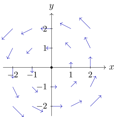
Figura 34.5: Campo vectorial \mathbf{F}(x, y) = (-y, x) : vectores tangentes a círculos concéntricos orientados en sentido antihorario ( \nabla \cdot \mathbf{F} = 0 ; \nabla \times \mathbf{F} = 2\mathbf{k} )
