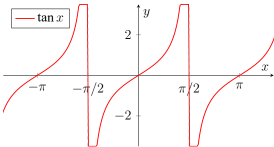
Figura 3.10: \text{tan } x : período \pi , asíntotas verticales en x = \pi/2 + k\pi .
