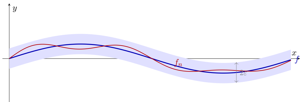
Figura 25.1: Convergencia uniforme f_n \Rightarrow f : para n suficientemente grande, la gráfica completa de f_n queda atrapada dentro de la banda de anchura 2\varepsilon alrededor de f . Un único N(\varepsilon) sirve para todos los x a la vez, y la banda se estrecha al hacer \varepsilon \rightarrow 0 .
