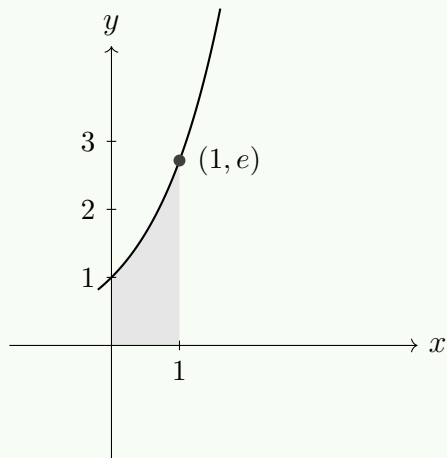
Figura 31.4: Lámina acotada por y = e^x , y = 0 , x = 0 , x = 1 con densidad \rho(x, y) = 2 - x + y .
