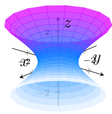
Figura 17.15: Hiperboloide de una hoja x^2 + y^2 - z^2 = 1 .
