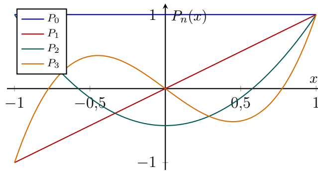
Figura 29.3: Polinomios de Legendre P_0, \dots, P_3 en [-1, 1] . Cada P_n tiene n ceros en el intervalo, satisface P_n(1) = 1 y tiene la paridad de n ; son mutuamente ortogonales.
