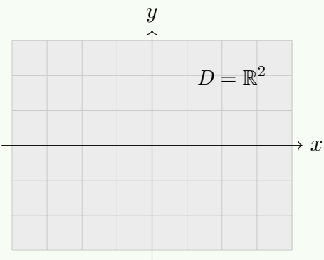
Figura 17.27: Dominio de f(x, y) = \ln(1 + 4x^2 + y^2) : todo \mathbb{R}^2
