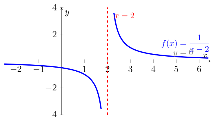
Figura 4.5: f(x) = 1/(x - 2) : asíntota vertical x = 2 (los valores crecen sin cota al acercarse a 2) y asíntota horizontal y = 0 (la función se aplanan hacia el eje x cuando x \rightarrow \pm\infty ).
