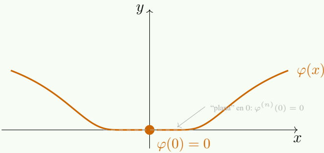
Figura 25.14: Función C^\infty que no es analítica en el origen: todas sus derivadas se anulan en 0, por lo que su serie de Taylor es idénticamente nula y no representa a la función en ningún entorno.
