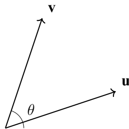
Figura 7.11: Ángulo entre vectores
