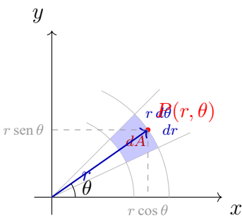
Figura 31.6: Coordenadas polares: el punto P satisface x = r \cos \theta, y = r \operatorname{sen} \theta ; el rectángulo polar (azul) tiene área dA = r \, dr \, d\theta
