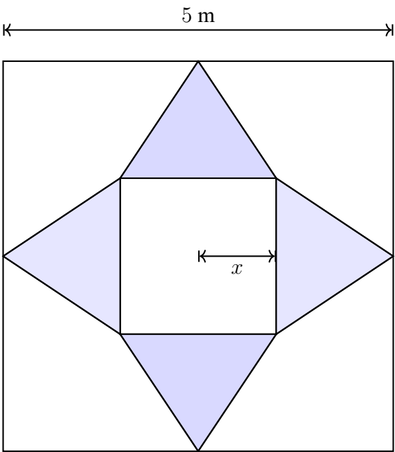
Figura 3.17: Patrón para la tienda de acampar (pirámide de base cuadrada): cuadrado de 5\text{ m} de lado; x es la distancia del centro al lado de la base.
