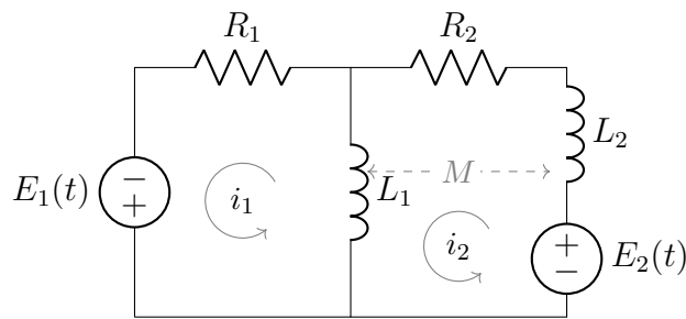
Figura 28.3: Circuito de dos mallas acopladas por inductancia mutua M . Las corrientes i_1(t), i_2(t) satisfacen L_1 i_1' + R_1 i_1 + M i_2' = E_1 y M i_1' + L_2 i_2' + R_2 i_2 = E_2 .
