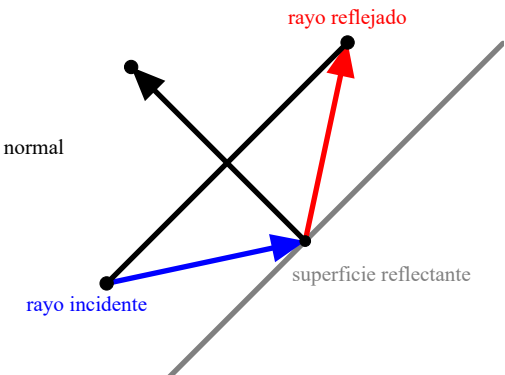
Figura 7.18: Rayo incidente, normal a la superficie reflectante y rayo reflejado en el punto de incidencia.
