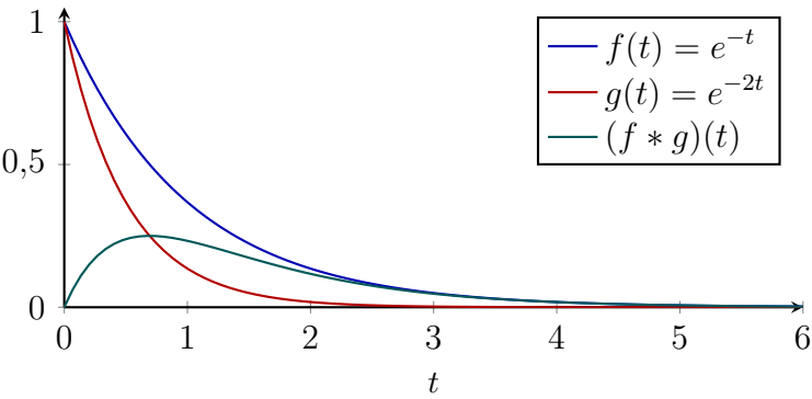
Figura 30.3: Convolución de f(t) = e^{-t} y g(t) = e^{-2t} : (f * g)(t) = \int_0^t f(\tau)g(t - \tau) d\tau = e^{-t} - e^{-2t} . El Teorema 30-39 la convierte en un producto, \mathcal{L}\{f * g\} = F(s)G(s) .
