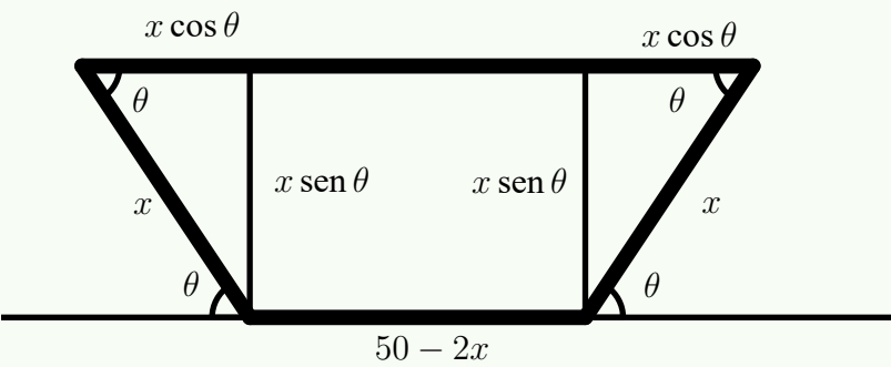
Figura 21.2: Sección transversal del canal abierto en forma de trapecio con ángulos iguales \theta en la base; x es la longitud del lado doblado.
