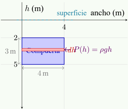
Figura 10.24: Compuerta rectangular sumergida entre las profundidades h = 2 m y h = 5 m. La presión crece linealmente con la profundidad, de modo que la fuerza se obtiene integrando franjas horizontales.
