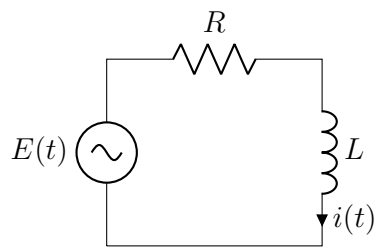
Figura 26.3: Circuito RL en serie con fuente de voltaje E(t) . La corriente i(t) satisface L i' + R i = E(t) .
