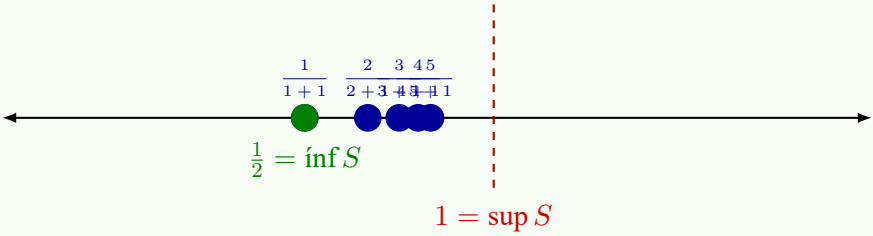
Figura 1.9: Los puntos \frac{n}{n+1} crecen hacia el supremo 1 sin alcanzarlo; el mínimo \frac{1}{2} , que es el ínfimo, sí pertenece a S .
