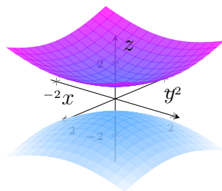
Figura 17.16: Hiperboloide de dos hojas z^2 - x^2 - y^2 = 1 .
