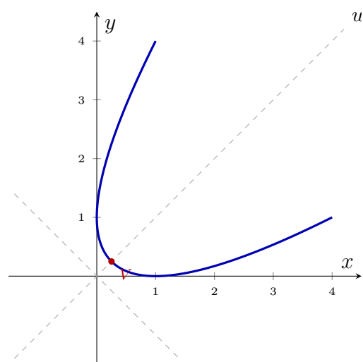
Figura 17.30: La cónica x^2 + y^2 - 2xy - 2(x + y) + 1 = 0 (azul) y los ejes girados u = x + y , v = x - y ; su vértice es V = (\frac{1}{4}, \frac{1}{4}) .
