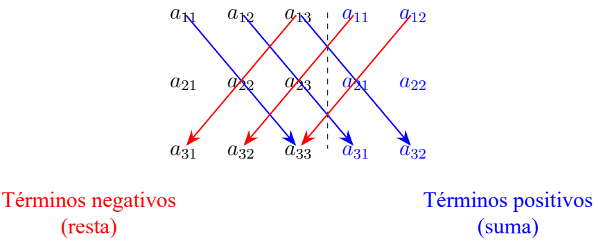
Figura 13.6: Regla de Sarrus, método de extender columnas
