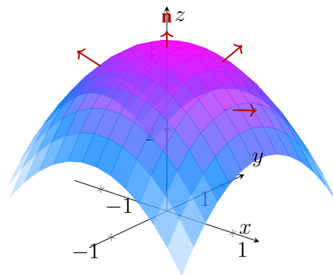
Figura 34.6: Superficie orientada z = 4 - x^2 - y^2 con vectores normales \mathbf{n} consistentes; invertir la orientación cambia el signo del flujo
