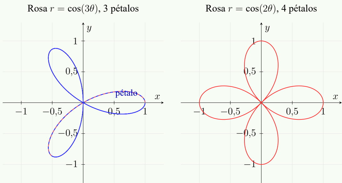
Figura 12.7: Rosas polares r = \cos(n\theta) : con n impar se obtienen n pétalos (aquí r = \cos 3\theta , 3 pétalos) y con n par se obtienen 2n pétalos (aquí r = \cos 2\theta , 4 pétalos).
