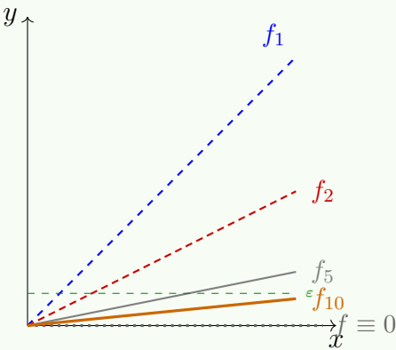
Figura 25.3: Sucesión de funciones lineales que converge uniformemente en [0, 1] : el error máximo \sup |f_n - f| tiende a cero al aumentar n .
