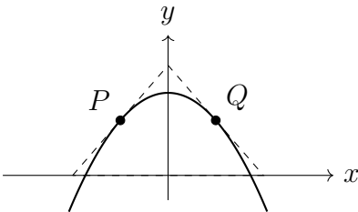
Figura 5.4: Triángulo equilátero formado por el eje x y las rectas tangentes.
