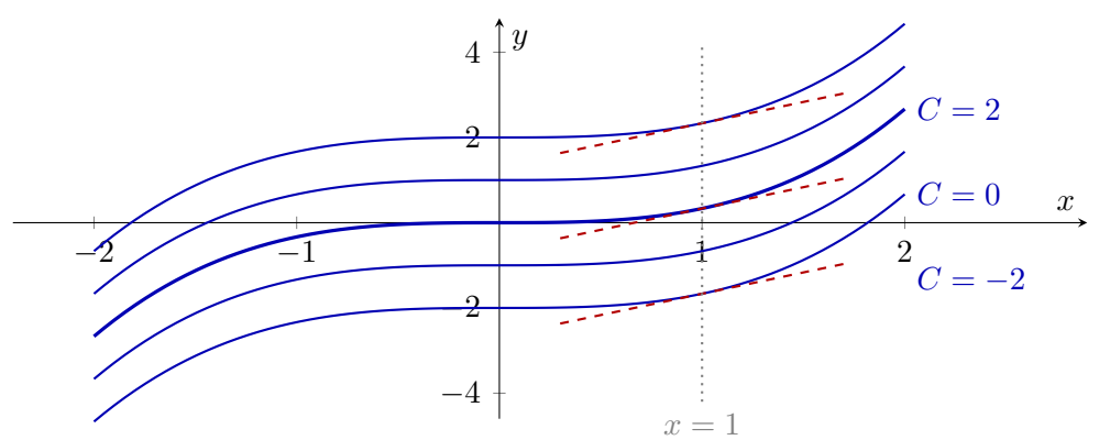
Figura 8.1: Familia de antiderivadas F(x) = \frac{x^3}{3} + C de f(x) = x^2 . Las curvas son traslaciones verticales unas de otras y sus rectas tangentes en un mismo x (aquí x = 1 , en rojo) son paralelas, pues todas tienen pendiente f(1) = 1 .
