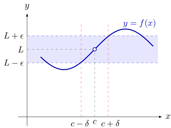
Figura 4.2: Definición \epsilon - \delta : fijada la tolerancia \epsilon alrededor de L (banda horizontal), existe \delta tal que todo x del entorno perforado (c - \delta, c + \delta) tiene imagen dentro de la banda. El valor f(c) , si existe, es irrelevante (punto excluido).
