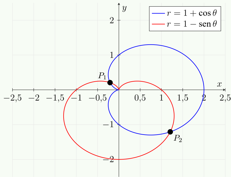
Figura 12.11: Dos cardioides, r = 1 + \cos \theta (hacia la derecha) y r = 1 - \operatorname{sen} \theta (hacia abajo): se cruzan en dos puntos y comparten el polo, lo que delimita la región común.
