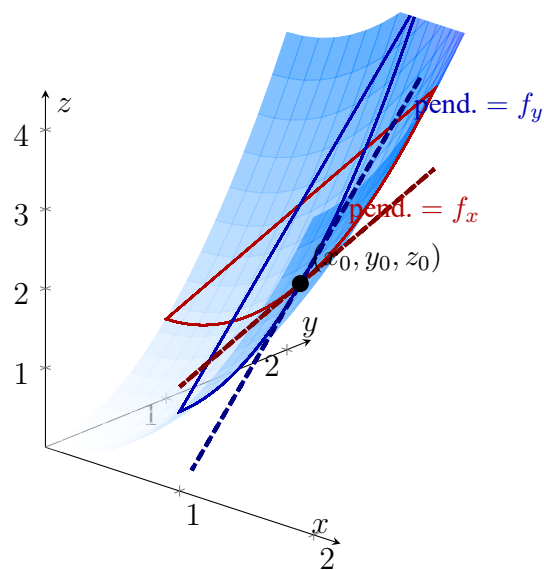
Figura 19.1: Interpretación geométrica de las derivadas parciales: la curva roja (corte y = y_0 ) tiene recta tangente (roja punteada) con pendiente f_x(x_0, y_0) ; la curva azul (corte x = x_0 ) tiene recta tangente (azul punteada) con pendiente f_y(x_0, y_0) .
