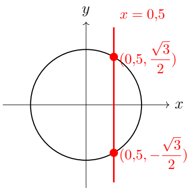
Figura 3.3: La circunferencia unitaria falla la prueba de la recta vertical.
