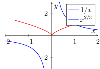
Figura 3.6: f(x) = 1/x con asíntota en x = 0 ( D_f = \mathbb{R} \setminus \{0\} ); g(x) = x^{2/3} con cúspide en el origen ( D_g = \mathbb{R} ).
