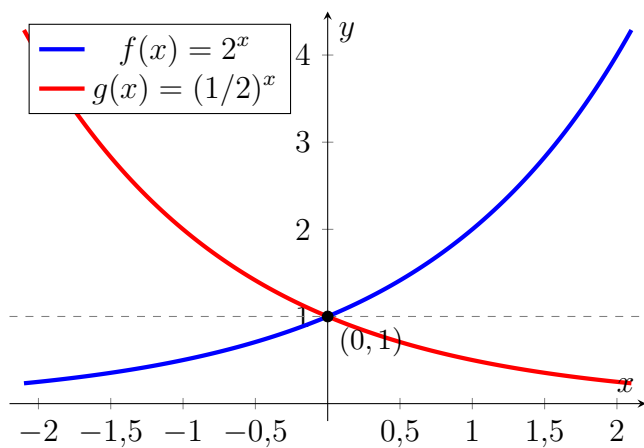
Figura 3.7: f(x) = 2^x creciente; g(x) = (1/2)^x decreciente. Ambas pasan por (0, 1) y tienen asíntota y = 0 .
