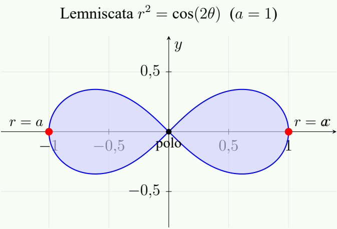
Figura 12.8: Lemniscata r^2 = a^2 \cos(2\theta) : dos bucles simétricos definidos donde \cos(2\theta) \geq 0 , con ancho máximo r = a en \theta = 0 .
