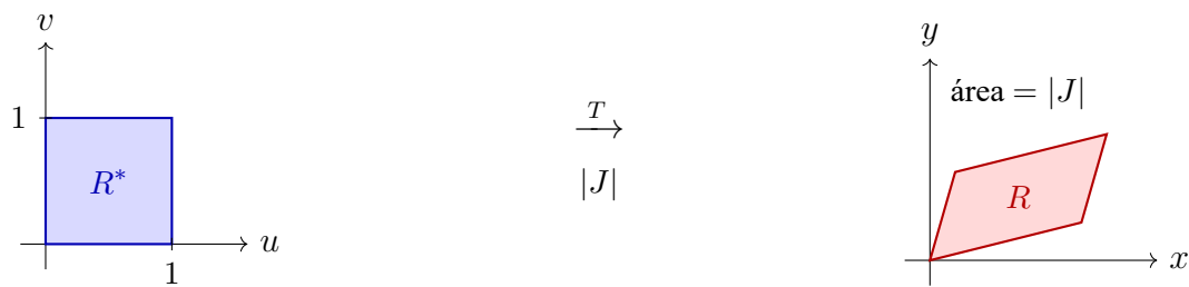
Figura 31.8: El jacobiano |J| es el factor de escala de área: el cuadrado R^* = [0, 1]^2 en (u, v) se transforma en la región R de área |J| en (x, y)
