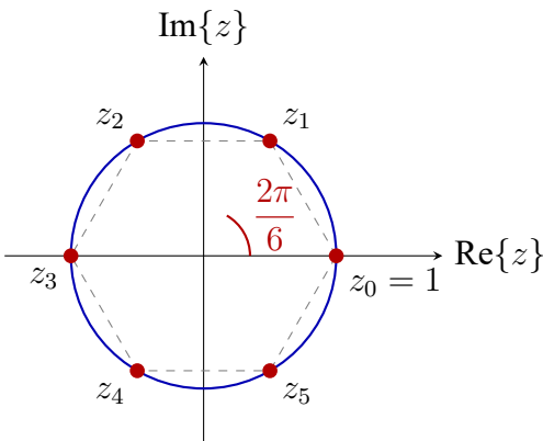
Figura 2.5: Las seis raíces sextas de la unidad ( z^6 = 1 ): todas tienen módulo 1 y sus argumentos \frac{2k\pi}{6} , con k = 0, \dots, 5 , difieren consecutivamente en \frac{2\pi}{6} , por lo que forman un hexágono regular inscrito en la circunferencia unitaria.
