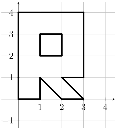
Figura 23.10: Figura original en el plano
