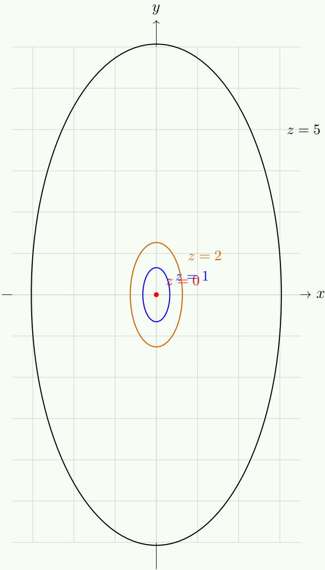
Figura 17.28: Curvas de nivel de f(x, y) = \ln(1 + 4x^2 + y^2) para z = 0, 1, 2, 5
