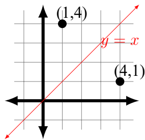
Figura 23.4: Reflexión respecto a la recta y = x .
