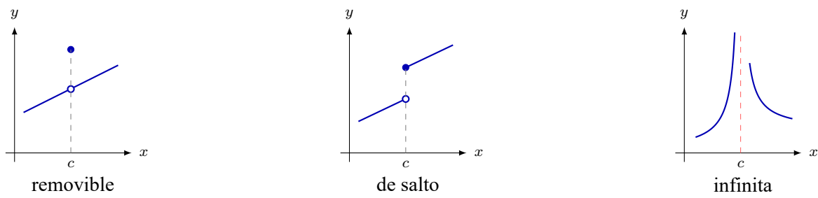
Figura 4.6: Tres tipos de discontinuidad en x = c : removible (el límite existe pero difiere de f(c) ), de salto (límites laterales distintos) e infinita (asíntota vertical).
