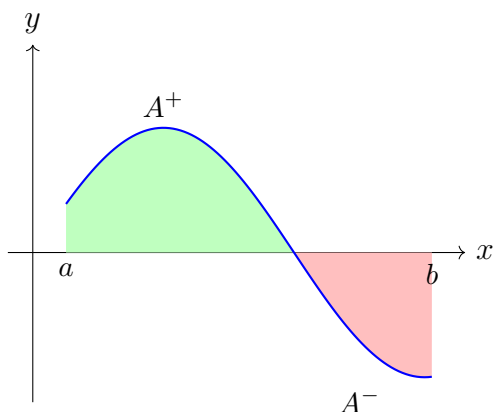
Figura 9.3: Interpretación de la integral definida como área neta : la región sobre el eje x (verde, A^+ ) aporta con signo positivo y la región bajo el eje (roja, A^- ) con signo negativo, de modo que \int_a^b f = A^+ - A^- .
