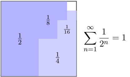
Figura 24.8: Demostración visual de \sum_{n=1}^{\infty} 2^{-n} = 1 : cada término cubre la mitad del área restante del cuadrado unitario ( \frac{1}{2} , luego \frac{1}{4} , \frac{1}{8} , ...), de modo que la unión de todos los rectángulos llena el cuadrado completo de área 1.
