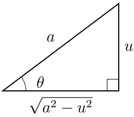
Figura 8.2: Triángulo de referencia del Caso 1, \sqrt{a^2 - u^2} . Con u = a \operatorname{sen} \theta el radical es el cateto adyacente, \sqrt{a^2 - u^2} = a \cos \theta .
