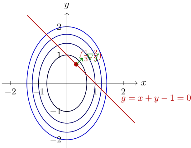
Figura 21.3: Método de Lagrange: el óptimo ocurre donde una curva de nivel de f (elipse azul) es tangente a la restricción g = 0 (recta roja); en ese punto \nabla f \parallel \nabla g
