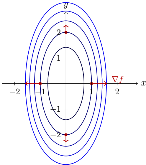
Figura 20.1: Curvas de nivel de f(x, y) = x^2 + \frac{y^2}{4} (elipses) con vectores \nabla f en cuatro puntos, perpendiculares a las curvas de nivel
