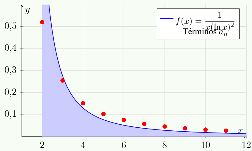
Figura 24.10: Términos a_n que decrecen lentamente ( a_{100} \approx 0,00217 ): el análisis gráfico sugiere convergencia, pero exige un criterio (integral o comparación) para confirmarla.
