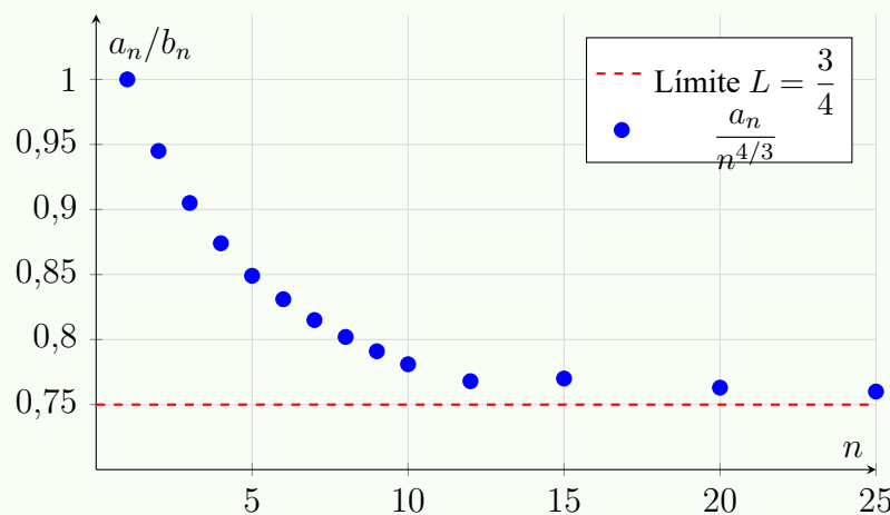
Figura 24.7: Cocientes a_n/b_n con a_n = \sum k^{1/3} y b_n = n^{4/3} : los valores 0,814, 0,789, 0,763, 0,758 sugieren convergencia a 3/4 (criterio de Stolz-Cesàro).
