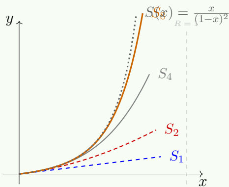
Figura 25.11: Suma en forma cerrada obtenida derivando término a término la serie geométrica: la operación es válida en el interior del intervalo de convergencia.
