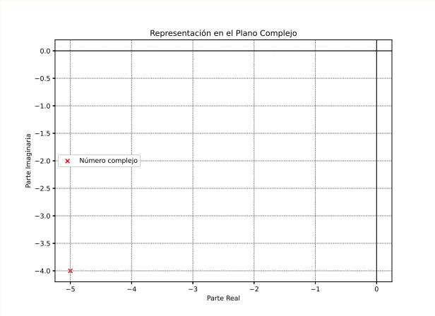
Figura 2.6: Representación gráfica en matplotlib del complejo -5 - 4i .
