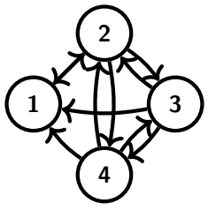
Figura 13.11: Grafo del ítem c)
