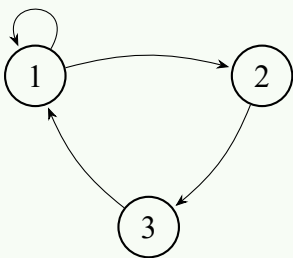
Figura 13.2: Grafo del ejemplo 13.13
