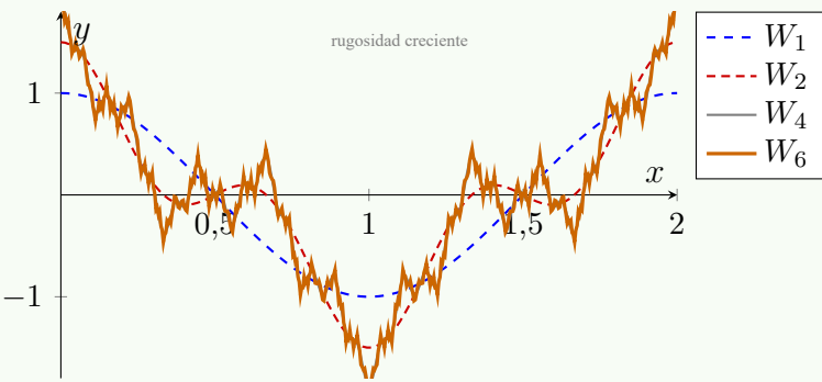
Figura 25.8: Función de Weierstrass: suma uniformemente convergente de cosenos con frecuencias crecientes, continua en todo punto pero derivable en ninguno por su estructura autosemejante.
