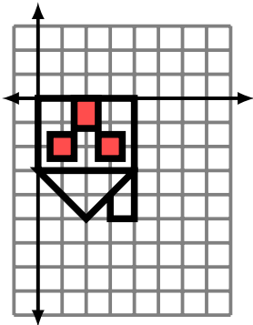
Figura 23.9: Reflexión de la casita respecto al eje x .
