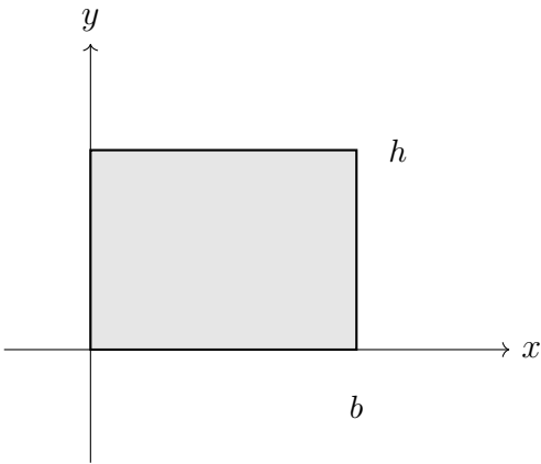
Figura 31.5: Lámina rectangular de ancho b y altura h con densidad uniforme \rho = 1 .
