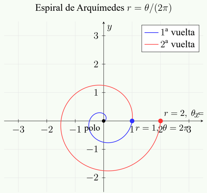
Figura 12.9: Espiral de Arquímedes r = a\theta : a diferencia de las curvas cerradas, se aleja indefinidamente del polo; con a = 1/(2\pi) cada vuelta aumenta r en una unidad.
