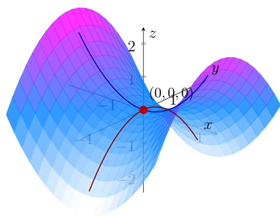
Figura 21.1: Punto de silla en el origen de z = x^2 - y^2 : curvatura positiva en dirección x (azul) y negativa en dirección y (rojo)
