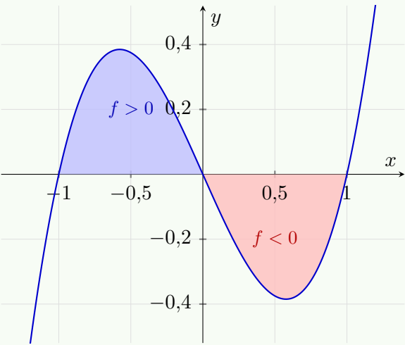
Figura 10.1: Región limitada por la curva y el eje x en [-1, 1] . El tramo situado sobre el eje (azul) aporta área positiva y el situado bajo el eje (rojo) aporta área negativa, de modo que el área geométrica exige integrar el valor absoluto en cada subintervalo.
