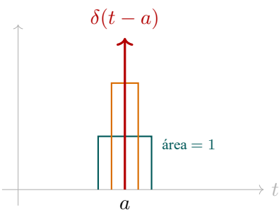
Figura 30.2: La delta de Dirac \delta(t - a) como límite de pulsos rectangulares de área 1: al estrecharse ( \epsilon \rightarrow 0^+ ) la altura crece manteniendo el área, concentrando toda la masa en t = a (flecha).
