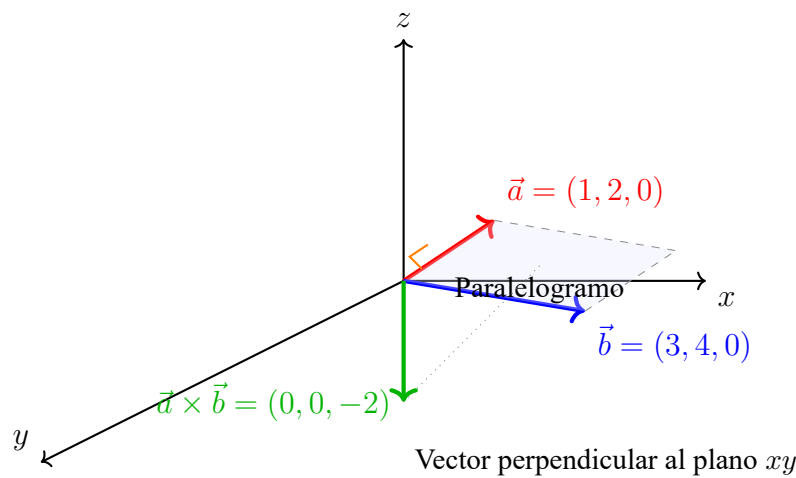
Figura 7.12: Producto cruz entre los vectores (1, 2, 0) y (3, 4, 0) . El resultado es un vector perpendicular al plano xy con dirección hacia el eje z negativo.
