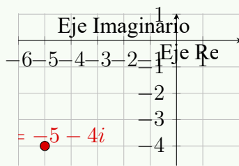
Figura 2.1: Representación geométrica del complejo -5 - 4i .
