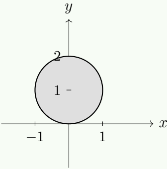
Figura 31.9: Lámina acotada por la curva polar r = 2 \operatorname{sen} \theta con densidad \rho(r, \theta) = r .
