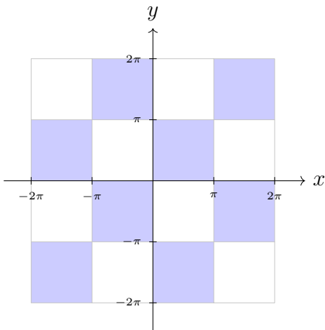
Figura 17.10: Dominio de f(x, y) = \sqrt{\sin x \sin y} (azul): tablero de cuadrados [k\pi, (k + 1)\pi] \times [m\pi, (m + 1)\pi] con k + m par, unidos por las rectas x = k\pi y y = m\pi .
