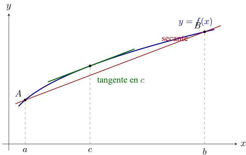
Figura 6.9: Teorema del Valor Medio: existe c \in (a, b) donde la recta tangente (verde) es paralela a la secante (roja) que une A = (a, f(a)) con B = (b, f(b)) ; en ese punto f'(c) = \frac{f(b) - f(a)}{b - a} .
