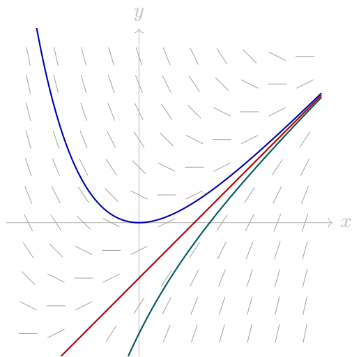
Figura 26.1: Campo de pendientes de y' = x - y con tres curvas solución y = x - 1 + Ce^{-x} ( C = 1, 0, -1 ). Todas convergen a la recta y = x - 1 ( C = 0 , en rojo) cuando x \rightarrow \infty .
