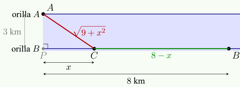
Figura 6.8: Tendido de tubería: cruce del río (ancho 3 km) desde A hasta el punto C a distancia x de P, y tramo terrestre C \rightarrow B de longitud 8 - x . El tramo submarino mide \sqrt{9 + x^2} .
