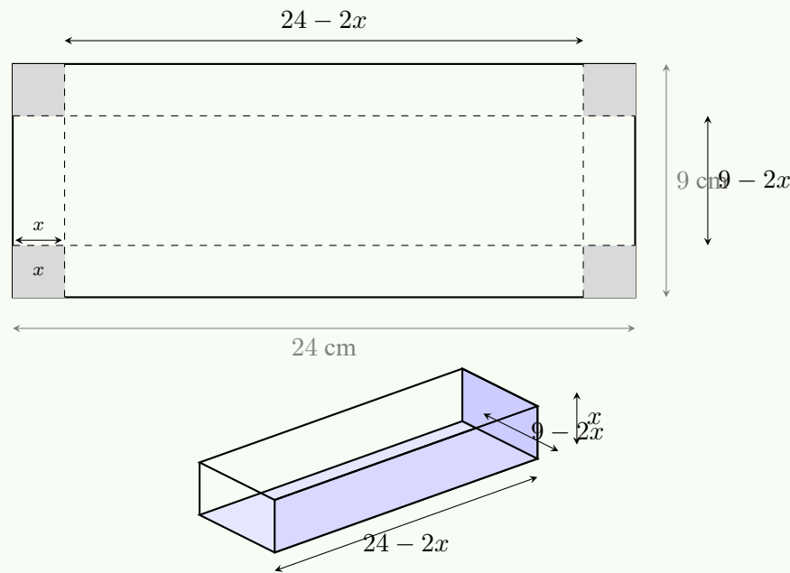
Figura 6.6: Construcción de la caja abierta: se recortan cuadrados de lado x en las esquinas de la lámina de 24 \times 9 cm y se doblan los bordes, quedando una base de (24 - 2x) \times (9 - 2x) y altura x .
