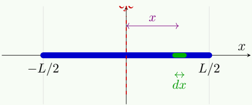
Figura 10.23: Misma varilla girando respecto a un eje que pasa por su centro: al situar el origen en el punto medio, la integral se extiende a [-L/2, L/2] y el momento de inercia resulta menor.
