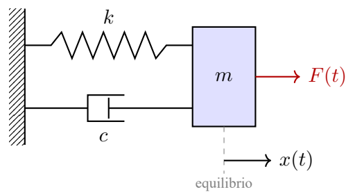
Figura 27.1: Sistema masa–resorte–amortiguador: masa m , constante del resorte k , coeficiente de amortiguamiento c y fuerza externa F(t) . El desplazamiento x(t) se mide desde la posición de equilibrio y satisface mx'' + cx' + kx = F(t) .
