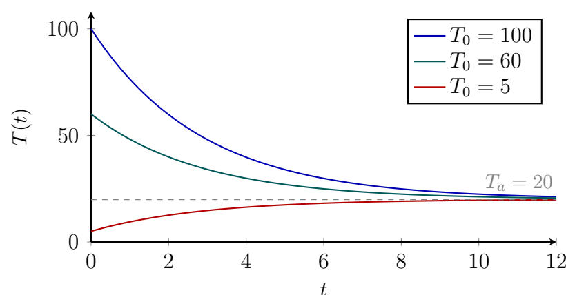
Figura 26.2: Ley de enfriamiento de Newton T(t) = T_a + (T_0 - T_a)e^{-kt} con T_a = 20 , k = 0,35 . Toda curva tiende asintóticamente a la temperatura ambiente; la de T_0 = 5 corresponde a un cuerpo que se calienta.
