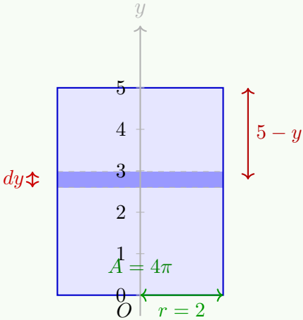
Figura 10.19: Tanque cilíndrico: a diferencia del cónico, la sección transversal es constante ( A = 4\pi \text{ m}^2 ) y solo varía la distancia de elevación 5 - y .
