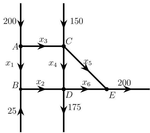
Figura 14.9: Flujos en una refinería de petróleo
