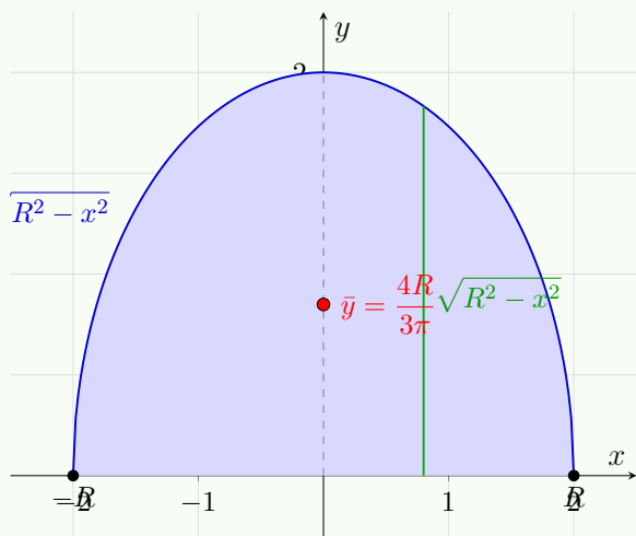
Figura 10.21: Lámina semicircular de radio R . La simetría respecto al eje y obliga a \bar{x} = 0 , de modo que solo hay que calcular \bar{y} .
