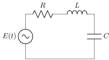
Figura 27.3: Circuito RLC en serie. La carga Q(t) del capacitor satisface LQ'' + RQ' + \frac{1}{C}Q = E(t) , análoga a mx'' + cx' + kx = F(t) con m \leftrightarrow L , c \leftrightarrow R , k \leftrightarrow 1/C .
