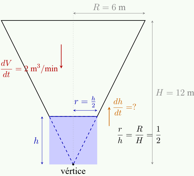
Figura 6.1: Corte transversal del tanque cónico invertido: por semejanza de triángulos, el radio de la superficie libre es proporcional a la profundidad h del agua.
