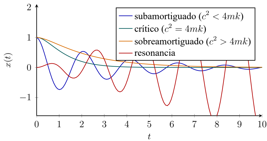
Figura 27.2: Los cuatro comportamientos del oscilador mx'' + cx' + kx = F(t) : subamortiguado (oscila y decae), crítico y sobreamortiguado (decaen sin oscilar), y resonancia (amplitud creciente cuando la forzante coincide con la frecuencia natural \omega_0 = \sqrt{k/m} ).
