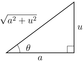
Figura 8.3: Triángulo de referencia del Caso 2, \sqrt{a^2 + u^2} . Con u = a \tan \theta el radical es la hipotenusa, \sqrt{a^2 + u^2} = a \sec \theta .
