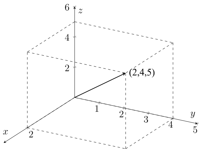
Figura 7.4: Vector \begin{pmatrix} 2 \\ 4 \\ 5 \end{pmatrix} en el espacio
