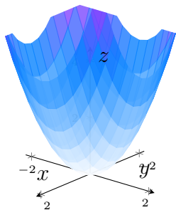
Figura 17.12: Paraboloide elíptico z = x^2 + y^2 .
