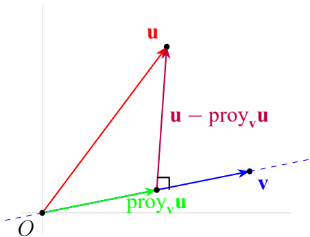
Figura 7.15: Proyección ortogonal del vector \mathbf{u} sobre el vector \mathbf{v} .
