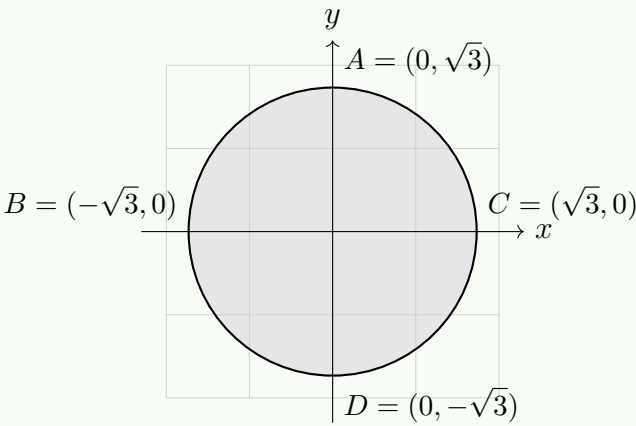
Figura 17.9: Dominio de f(x, y) = \sqrt{-3x^2 - 3y^2 + 9} : disco x^2 + y^2 \leq 3
