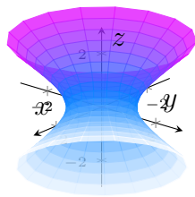
Figura 17.15: Hiperboloide de una hoja x^2 + y^2 - z^2 = 1 .
