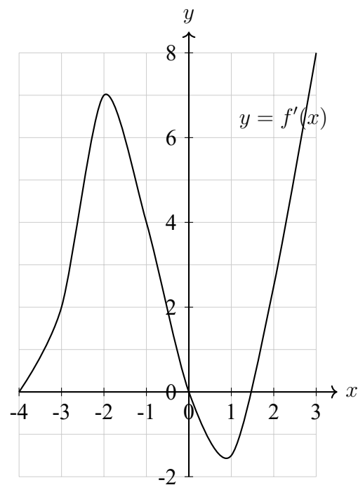
Figura 6.13: Gráfica de la derivada f' : los ceros de f' señalan los posibles extremos de f , el signo de f' su monotonía, y el crecimiento o decrecimiento de f' la concavidad de f .
