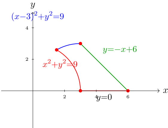
Figura 31.12: Región del segundo ejercicio
