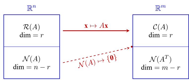
Figura 15.3: Esquema de los espacios fundamentales de A \in \mathcal{M}_{m \times n}(\mathbb{R}) con \text{rango}(A) = r . En el dominio \mathbb{R}^n conviven el espacio fila ( \dim r ) y el espacio nulo ( \dim n - r ), que satisfacen el teorema del rango-nulidad r + (n - r) = n ; la matriz envía el espacio fila sobre el espacio columna y aplasta el espacio nulo en \mathbf{0} .
