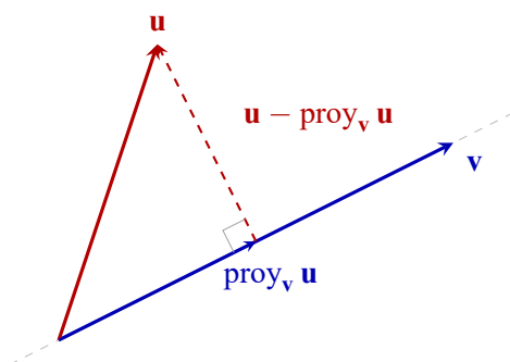
Figura 16.1: Proyección ortogonal de \mathbf{u} sobre \mathbf{v} : el vector \text{proy}_{\mathbf{v}} \mathbf{u} vive en la recta generada por \mathbf{v} y la diferencia \mathbf{u} - \text{proy}_{\mathbf{v}} \mathbf{u} es ortogonal a \mathbf{v} .
