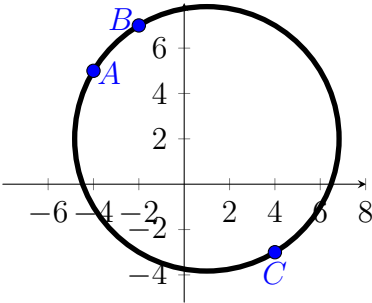
Figura 14.7: Circunferencia del problema
