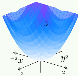
Figura 17.24: Familia de paraboloides z = x^2 + y^2 - k : k = 0 vértice en z = 0 (abajo) y k = -1 vértice en z = 1 (arriba).
