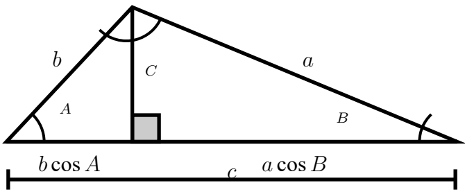
Figura 14.6: Triángulo del problema
