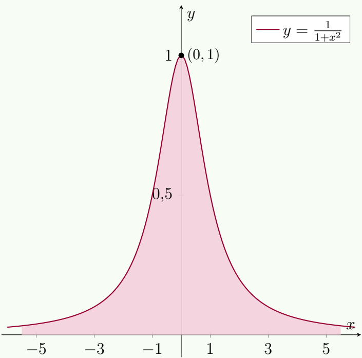
Figura 11.3: La función par f(x) = \frac{1}{1+x^2} con máximo f(0) = 1 y asíntota horizontal y = 0 . La región bajo la curva se extiende infinitamente a ambos lados, por lo que la integral se parte en c = 0 .
