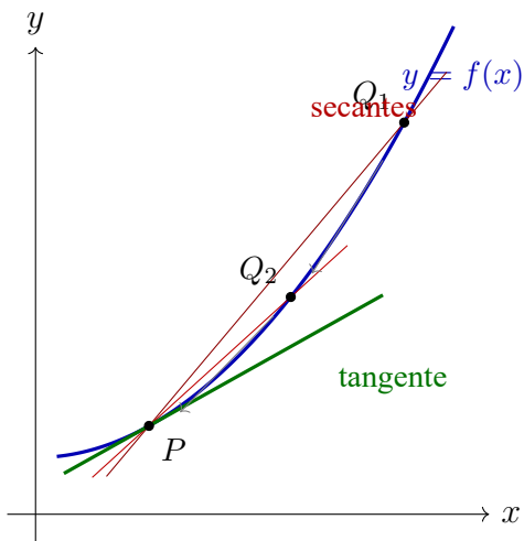
Figura 5.1: La recta secante por P = (x_0, f(x_0)) y un punto Q = (x_0 + h, f(x_0 + h)) tiende a la recta tangente en P cuando Q \rightarrow P (es decir, h \rightarrow 0 ); su pendiente \frac{f(x_0 + h) - f(x_0)}{h} tiende a f'(x_0) .
