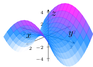
Figura 17.13: Paraboloide hiperbólico z = x^2 - y^2 (silla de montar).
