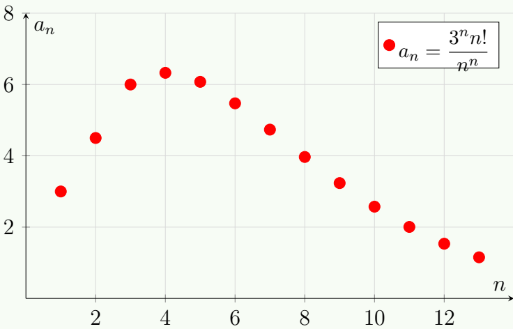
Figura 24.11: Términos con n! y n^n que crecen y luego decrecen: la presencia de factoriales y potencias hace idóneo el criterio del cociente.
