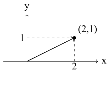
Figura 7.3: Vector \begin{pmatrix} 2 \\ 1 \end{pmatrix} en el plano
