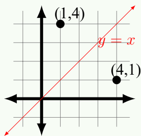
Figura 23.11: Reflexión respecto a la recta y = x .
