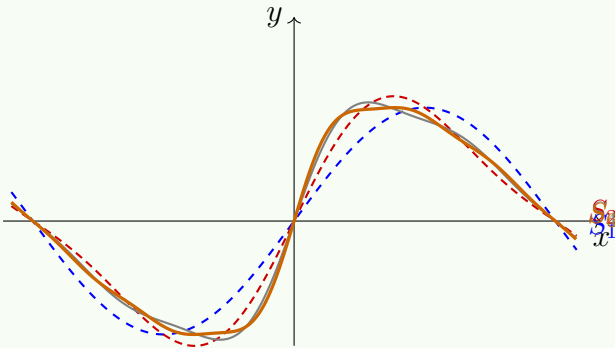
Figura 25.6: Serie trigonométrica cuya convergencia uniforme se establece con el criterio-M de Weierstrass: las sumas parciales se aproximan uniformemente a la función suma, continua e integrable.
