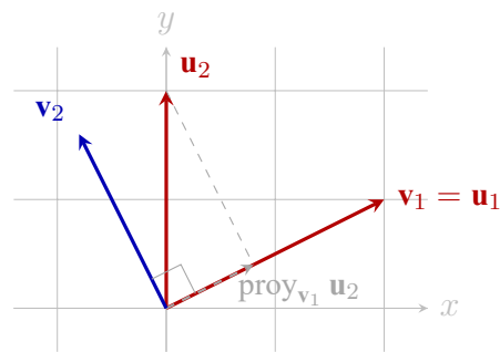
Figura 16.2: Proceso de Gram-Schmidt en \mathbb{R}^2 : de la base \{\mathbf{u}_1, \mathbf{u}_2\} se obtiene la base ortogonal \{\mathbf{v}_1, \mathbf{v}_2\} tomando \mathbf{v}_1 = \mathbf{u}_1 y restando de \mathbf{u}_2 su proyección sobre \mathbf{v}_1 : \mathbf{v}_2 = \mathbf{u}_2 - \text{proy}_{\mathbf{v}_1} \mathbf{u}_2 .
