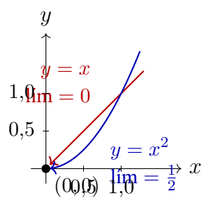
Figura 18.2: Dos trayectorias hacia (0,0) producen límites distintos para f(x,y) = \frac{x^2y}{x^4+y^2}
