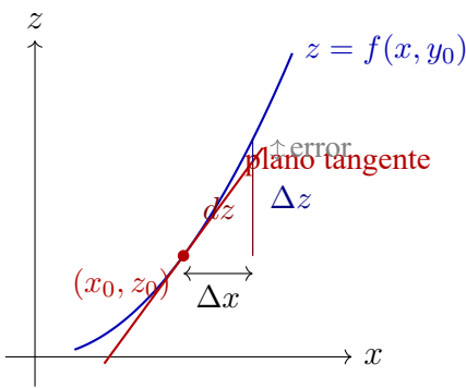
Figura 19.3: Aproximación lineal: dz (plano tangente) aproxima \Delta z (cambio real en la superficie) para incrementos pequeños \Delta x
