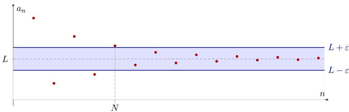
Figura 24.2: Convergencia de una sucesión: a_n \rightarrow L significa que para cada margen \varepsilon > 0 existe un umbral N tal que todos los términos con n > N caen dentro de la banda (L - \varepsilon, L + \varepsilon) . Solo un número finito de términos (los de índice n \leq N ) puede quedar fuera.
