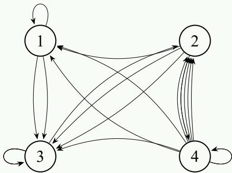
Figura 13.14: Grafo del problema (c)
