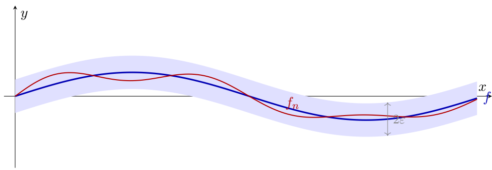
Figura 25.1: Convergencia uniforme f_n \Rightarrow f : para n suficientemente grande, la gráfica completa de f_n queda atrapada dentro de la banda de anchura 2\varepsilon alrededor de f . Un único N(\varepsilon) sirve para todos los x a la vez, y la banda se estrecha al hacer \varepsilon \rightarrow 0 .
