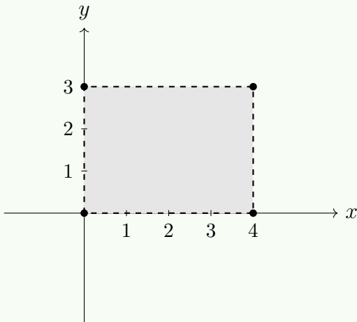
Figura 31.3: Lámina rectangular [0, 4] \times [0, 3] con densidad \rho(x, y) = y + 1 .
