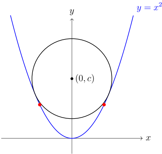
Figura 5.3: Un círculo de radio r inscrito en la parábola y = x^2 .
