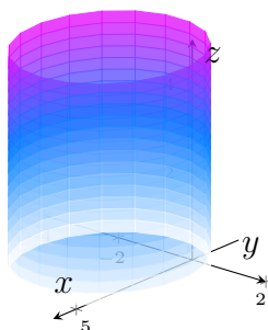
Figura 17.18: Cilindro elíptico \frac{(x - 2)^2}{9} + \frac{(y + 1)^2}{4} = 1 , con generatrices paralelas al eje z .
