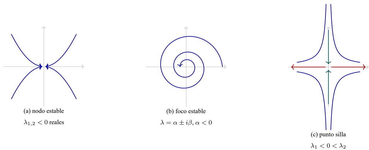
Figura 28.1: Retratos de fase de \mathbf{X}' = \mathbf{A}\mathbf{X} según el espectro de A : (a) nodo —valores propios reales del mismo signo, trayectorias que entran (o salen) del origen; (b) foco —valores propios complejos, espiral; (c) punto silla —valores propios reales de signo opuesto, con separatrices estable (verde, entra) e inestable (roja, sale).
