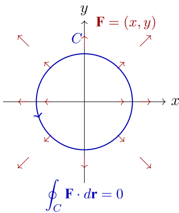
Figura 33.2: Campo conservativo \mathbf{F}(x, y) = (x, y) = \nabla\left(\frac{x^2+y^2}{2}\right) : las flechas apuntan radialmente; la integral sobre cualquier curva cerrada C es cero
