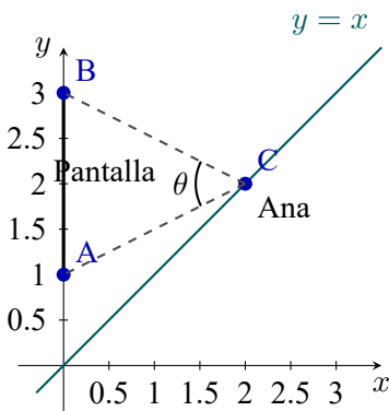
Figura 6.15: Ángulo de visión \theta de la pantalla AB (segmento vertical entre A(0, 1) y B(0, 3) ) desde un asiento C = (x, x) sobre la recta y = x .
