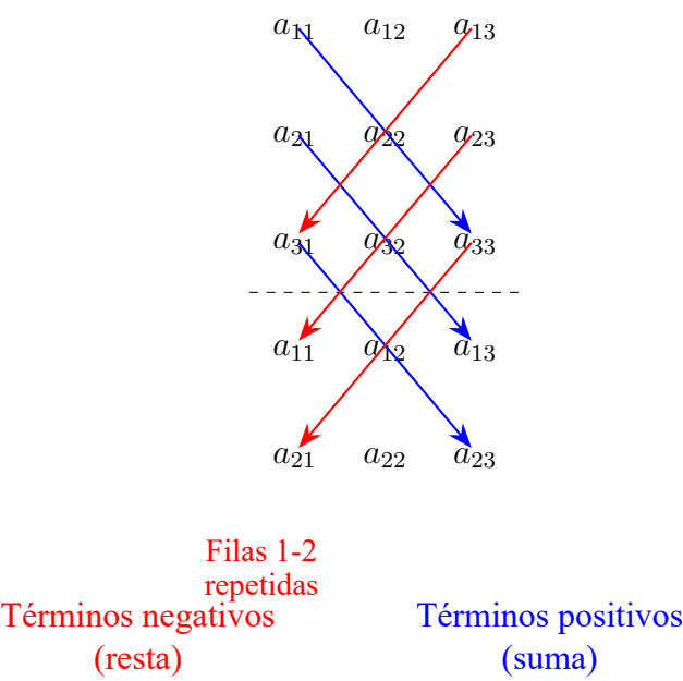
Figura 13.7: Regla de Sarrus, método de extender las filas
