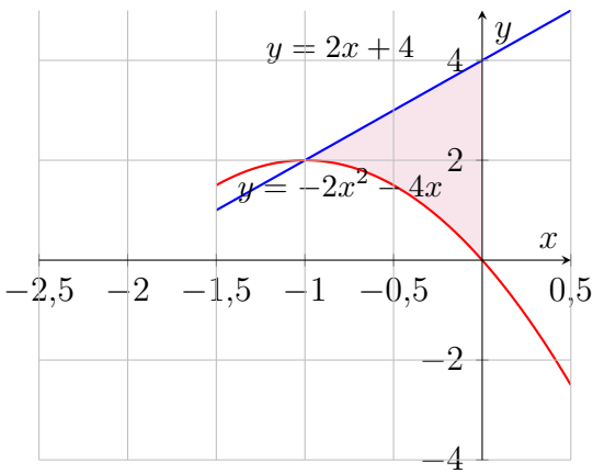
Figura 10.26: Región encerrada por y = 2x + 4 , y = -2x^2 - 4x y x = 0 , que se hace girar alrededor del eje x .
