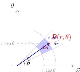
Figura 31.6: Coordenadas polares: el punto P satisface x = r \cos \theta, y = r \sin \theta ; el rectángulo polar (azul) tiene área dA = r \, dr \, d\theta
