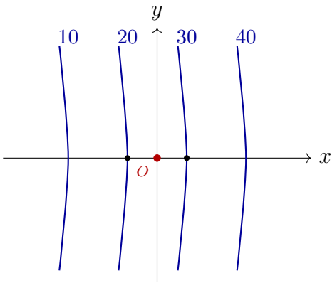
Figura 18.3: Mapa de contorno de f : las curvas de nivel 10, 20, 30, 40 cortan el eje x en x \approx -1,5, -0,5, 0,5, 1,5 . El origen O queda entre los niveles 20 y 30.
