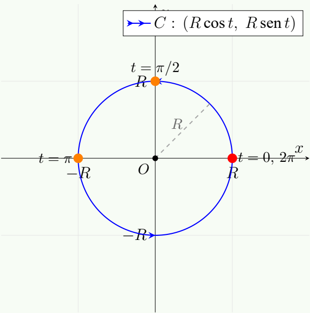
Figura 12.3: Circunferencia de radio R centrada en el origen, parametrizada y recorrida en sentido antihorario al crecer t (se ilustra con R = 1 ).
