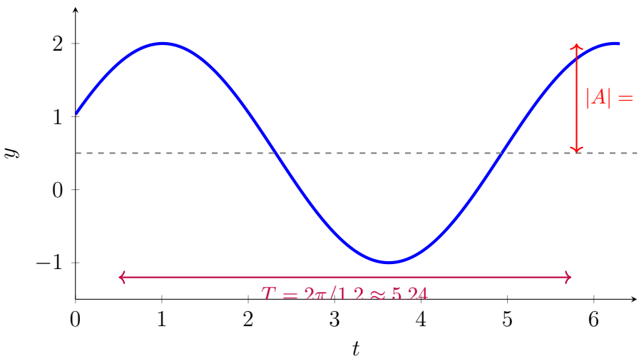
Figura 3.12: Parámetros de la forma amplitud-fase en y = C + A \operatorname{sen}[a(t - b)] .
