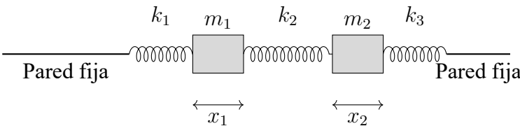
Figura 28.2: Dos masas m_1, m_2 acopladas por tres resortes ( k_1, k_2, k_3 ) entre paredes fijas. Los desplazamientos x_1, x_2 desde el equilibrio satisfacen un sistema lineal de segundo orden acoplado.
