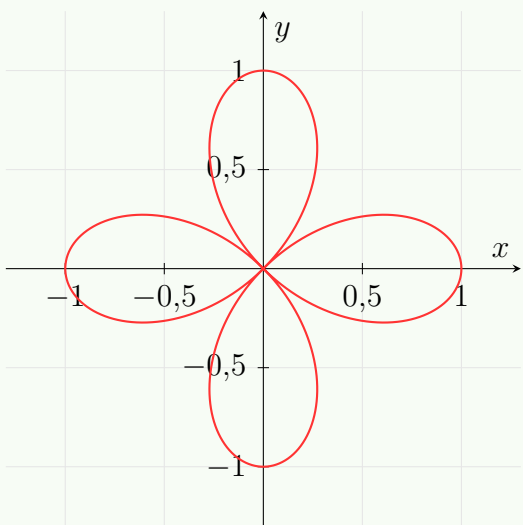
Rosa r = \cos(2\theta) , 4 pétalos
