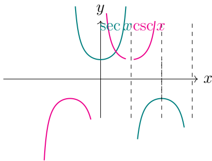
Figura 3.15: \sec x = 1/\cos x , \csc x = 1/\sin x : rango \mathbb{R} \setminus (-1, 1) , asíntotas verticales.
